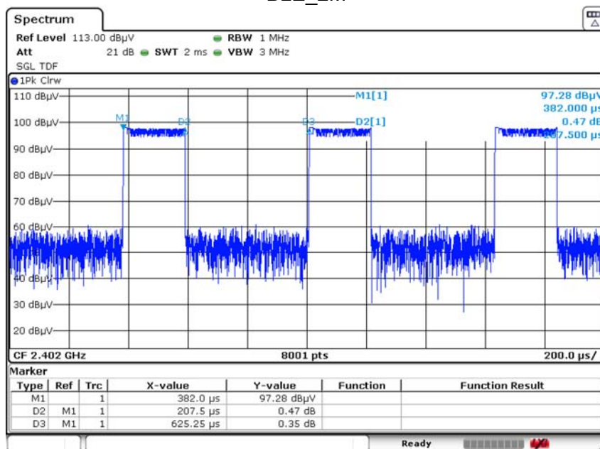
BLE_2M
