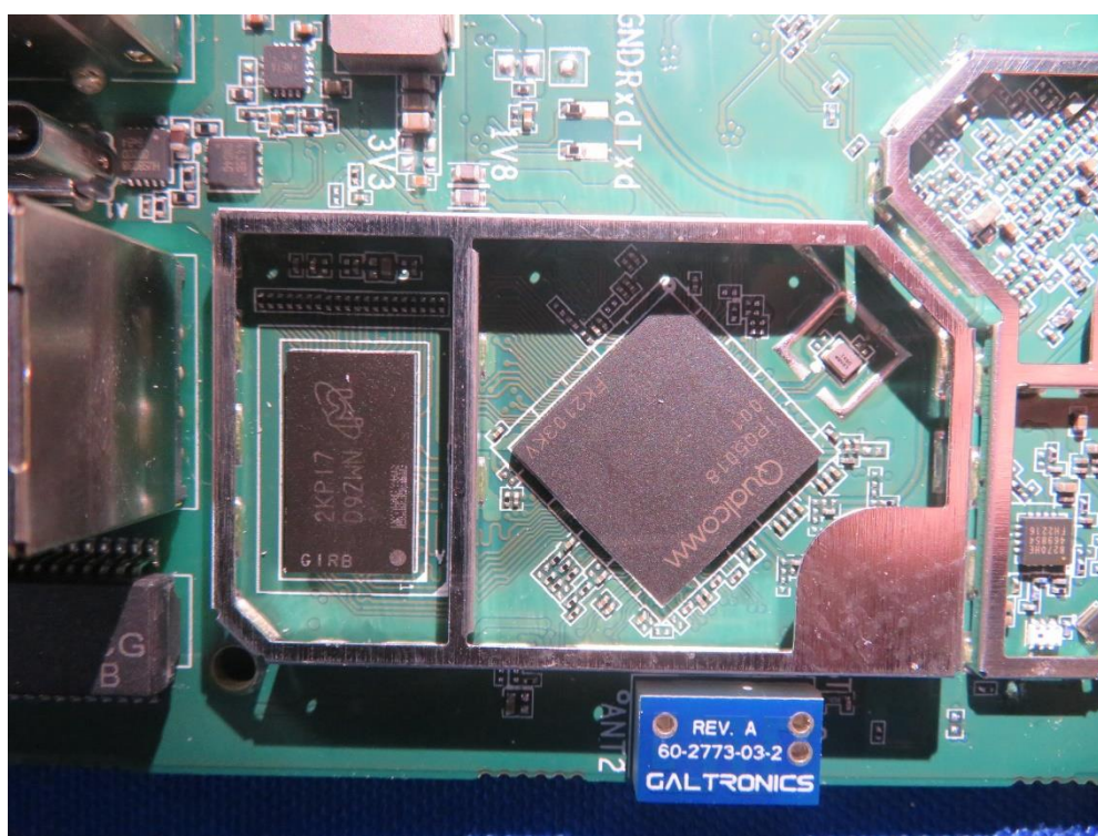
(14) EUT Photo
