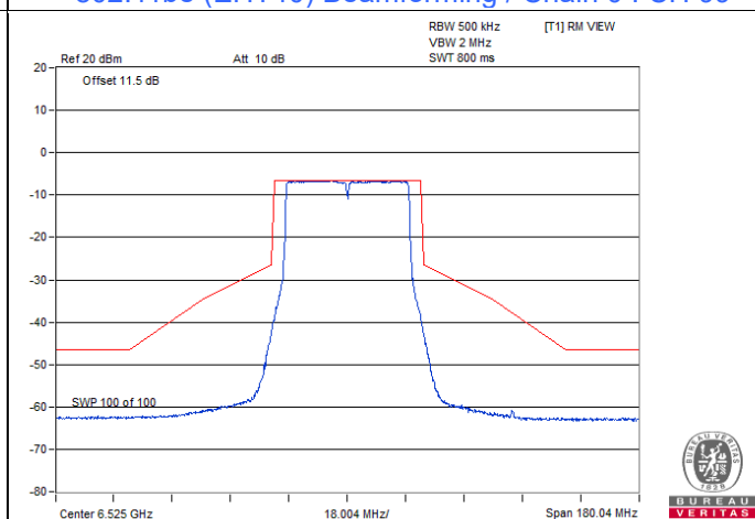
802.11be (EHT40) Beamforming / Chain 0 : CH 115
