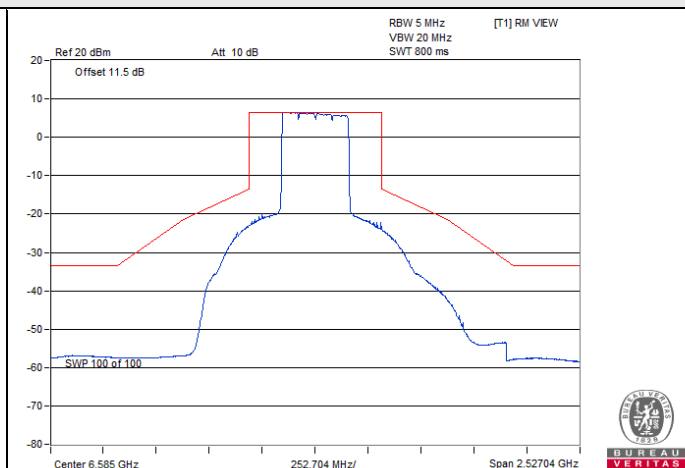
802.11be (EHT320) Beamforming / Chain 1 : CH 127
