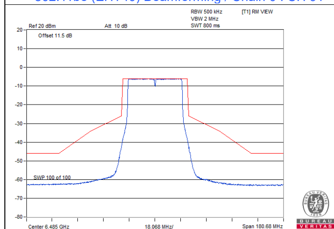
802.11be (EHT40) Beamforming / Chain 0 : CH 107
