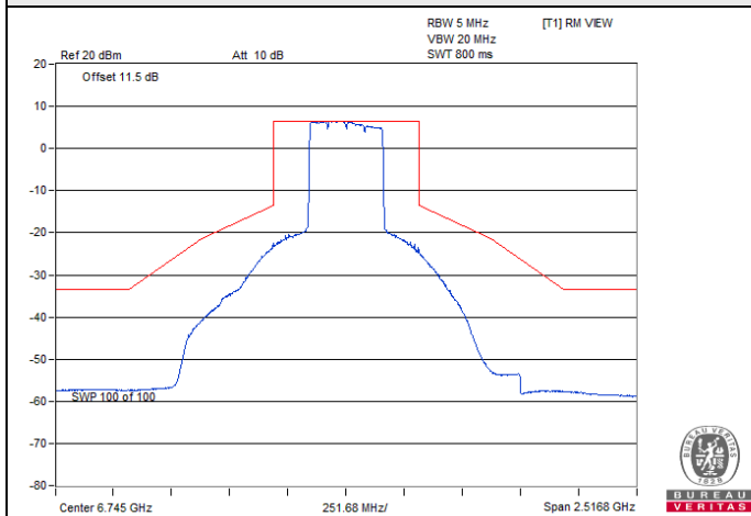
802.11be (EHT320) Beamforming / Chain 3 : CH 159
