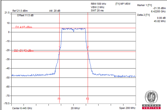
802.11be (EHT40) Beamforming / Chain 0 : CH 99
