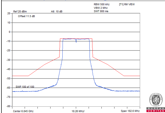
802.11be (EHT40) Beamforming / Chain 0 : CH 179
