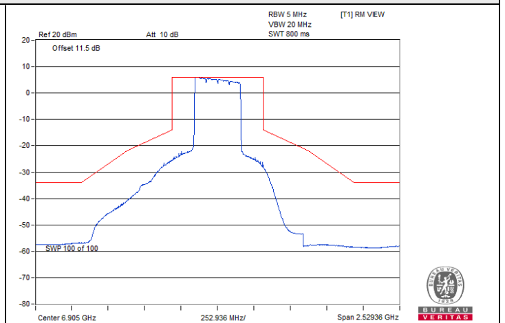
802.11be (EHT320) Beamforming / Chain 3 : CH 191
