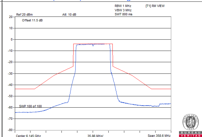
802.11be (EHT80) Beamforming / Chain 3 : CH 39
