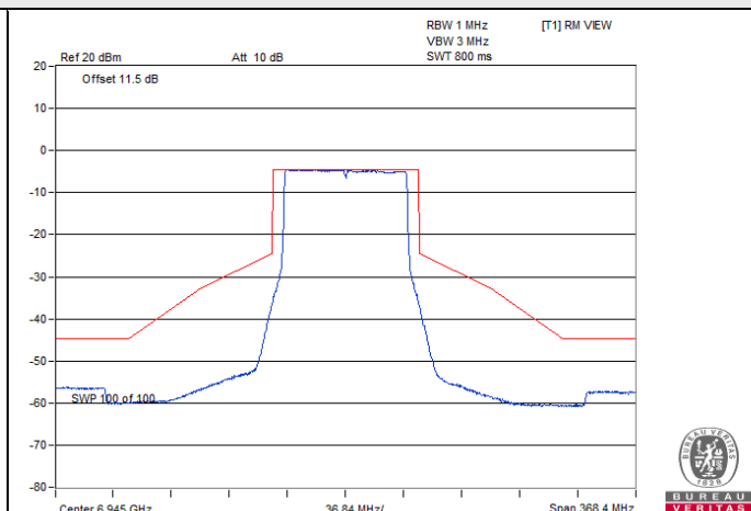
802.11be (EHT80) Beamforming / Chain 2 : CH 199
