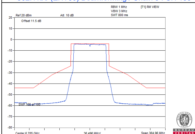
802.11be (EHT80) Beamforming / Chain 3 : CH 167
