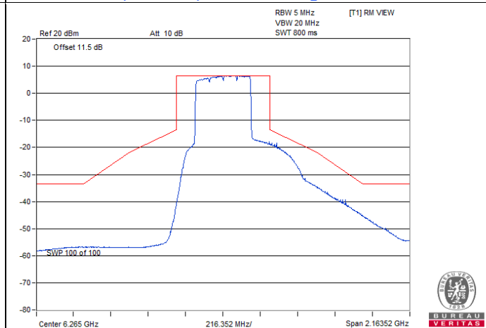
802.11be (EHT320) Beamforming / Chain 3 : CH 63
