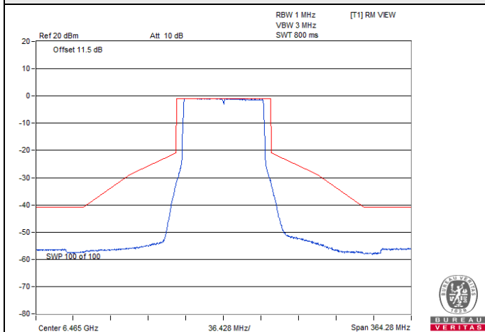
802.11be (EHT80) Beamforming / Chain 3 : CH 103
