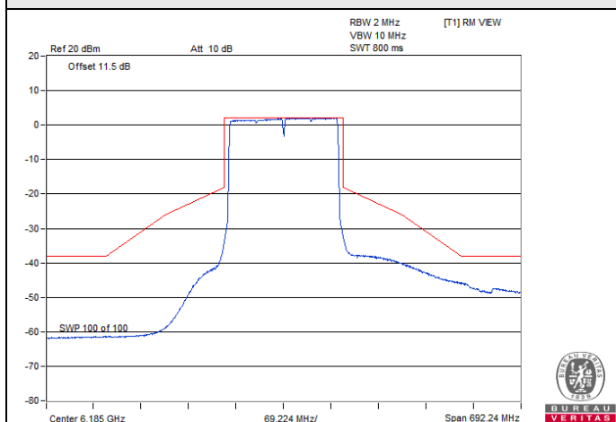
802.11be (EHT160) Beamforming / Chain 2 : CH 47
