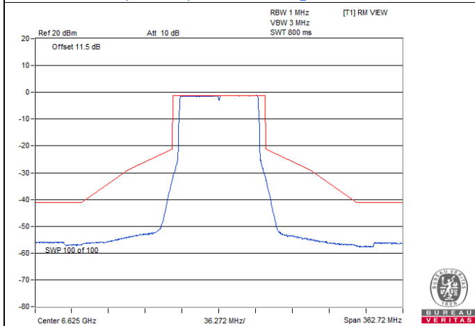
802.11be (EHT80) Beamforming / Chain 3 : CH 135
