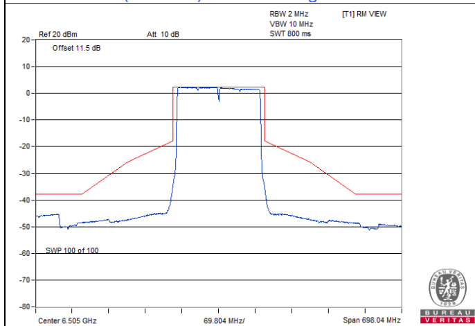
802.11be (EHT160) Beamforming / Chain 2 : CH 111
