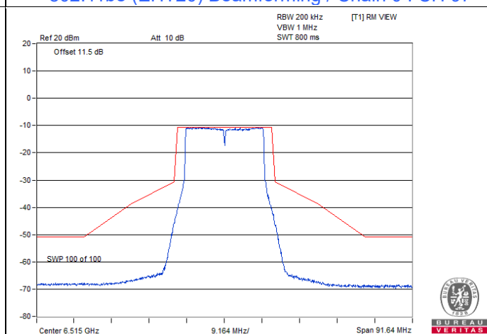
802.11be (EHT20) Beamforming / Chain 0 : CH 113
