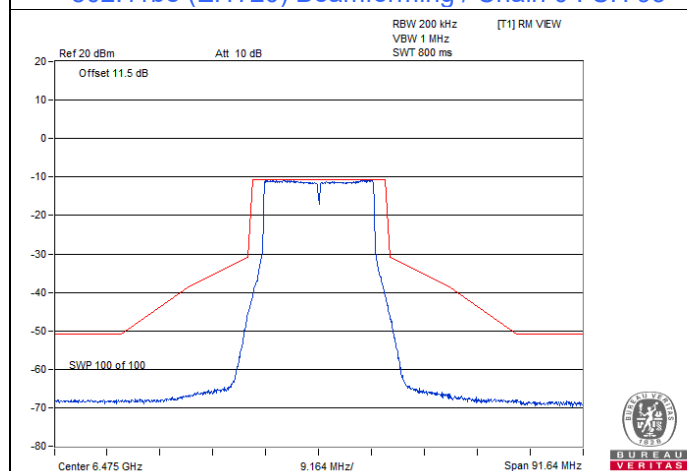
802.11be (EHT20) Beamforming / Chain 0 : CH 105
