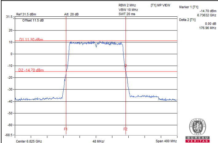
802.11be (EHT160) Beamforming / Chain 0 : CH 175
