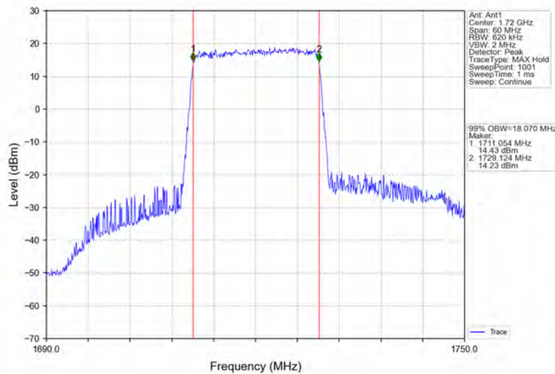
Band4_20MHz_QPSK_LCH_1720MHz_RB_100_0_NTNV
