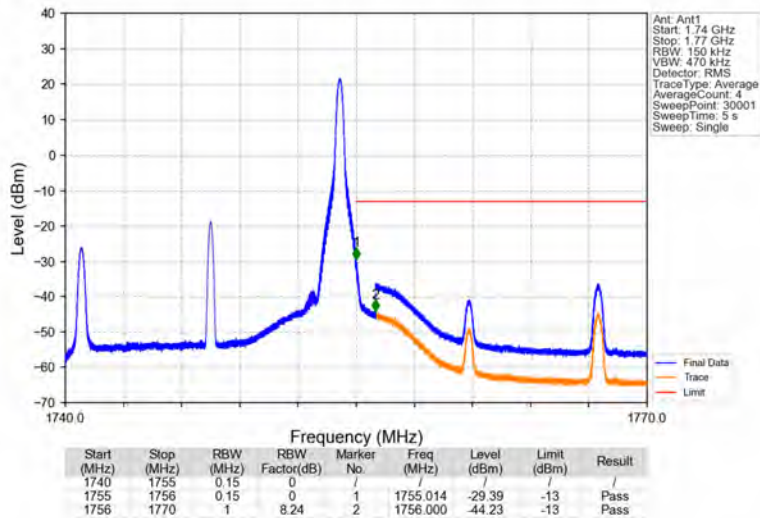
Band4_15MHz_QPSK_HCH_1747.5MHz_RB_1_74_NTNV
