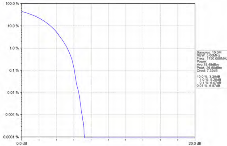
Band4_10MHz_QPSK_HCH_1750MHz_RB_50_0_NTNV
