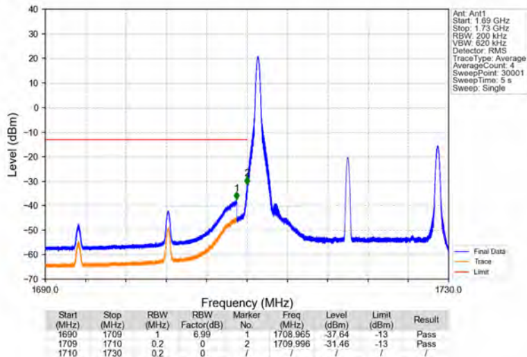
Band4_20MHz_16QAM_LCH_1720MHz_RB_1_0_NTNV
