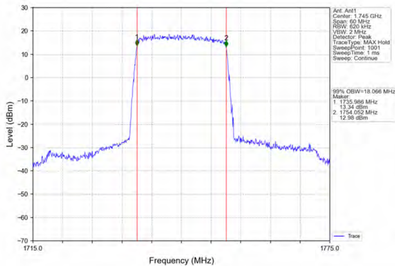
Band4_20MHz_QPSK_HCH_1745MHz_RB_100_0_NTNV
