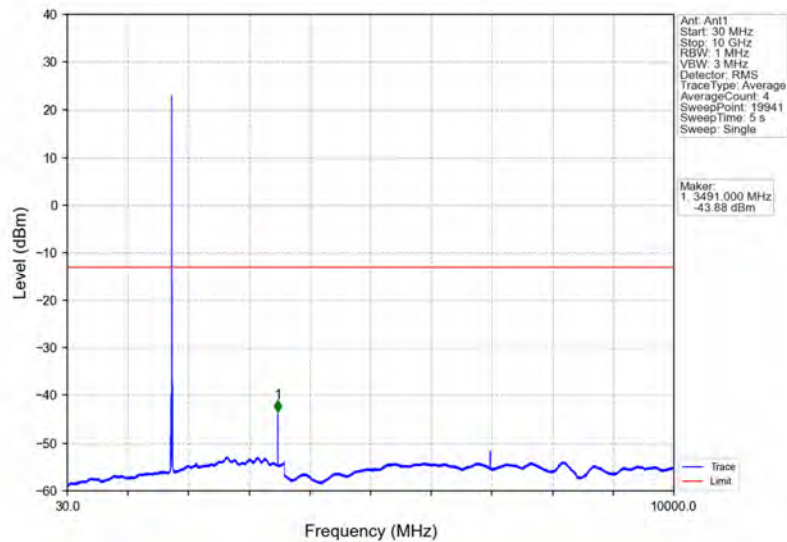
Band4_10MHz_QPSK_HCH_1750MHz_RB_1_0_NTNV
