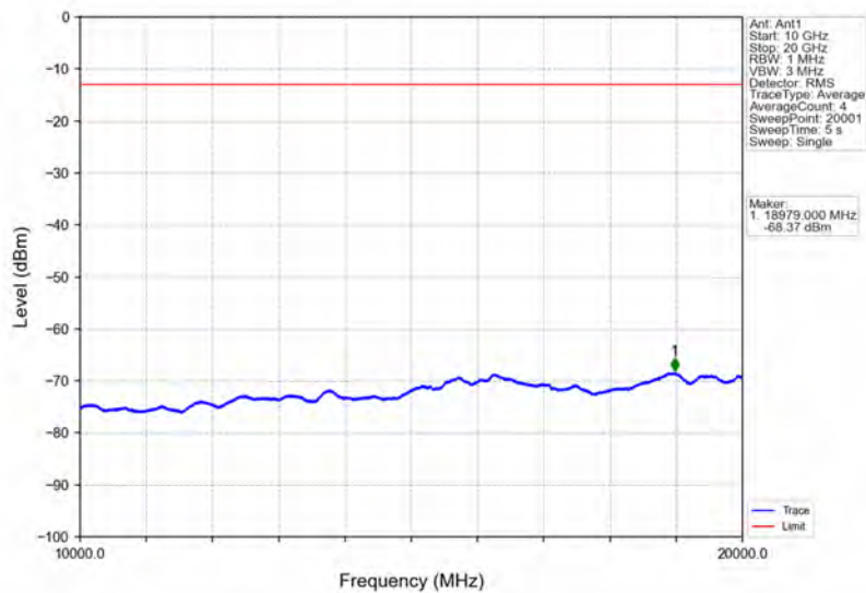
Band4_20MHz_QPSK_HCH_1745MHz_RB_1_0_NTNV
