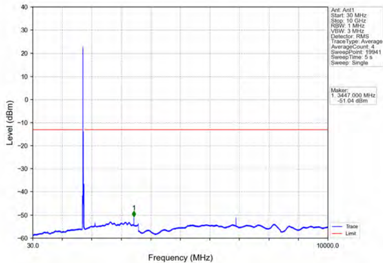
Band4_20MHz_QPSK_MCH_1732.5MHz_RB_1_0_NTNV
