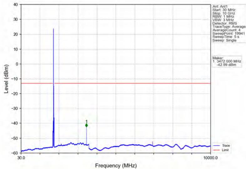
Band4_20MHz_QPSK_HCH_1745MHz_RB_1_0_NTNV
