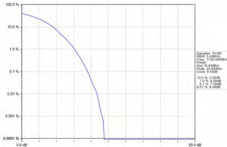
Band4_20MHz_16QAM_LCH_1720MHz_RB_100_0_NTNV
