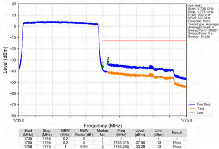
Band4_20MHz_QPSK_HCH_1745MHz_RB_100_0_NTNV
