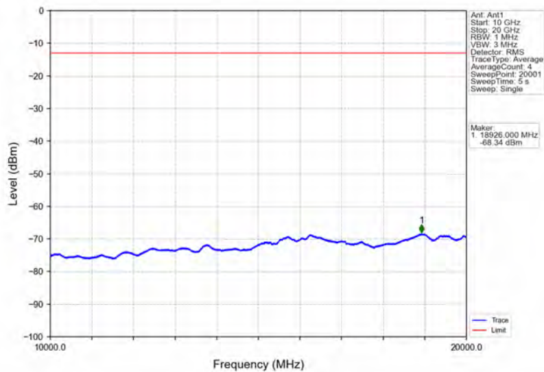
Band4_20MHz_QPSK_MCH_1732.5MHz_RB_1_0_NTNV
