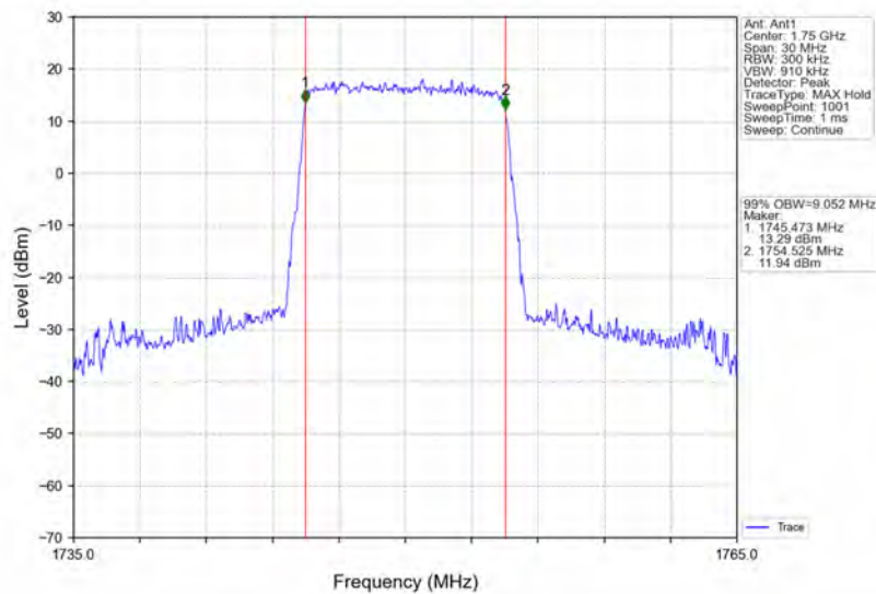
Band4_10MHz_QPSK_HCH_1750MHz_RB_50_0_NTNV
