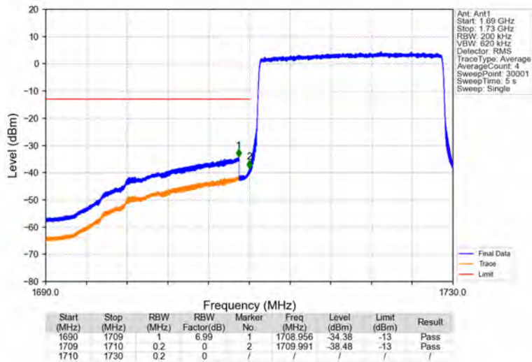
Band4_20MHz_16QAM_LCH_1720MHz_RB_100_0_NTNV
