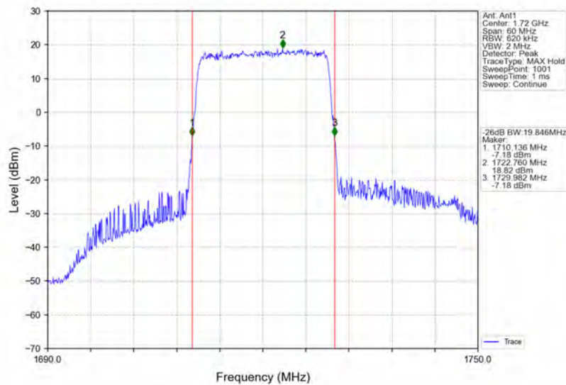
Band4_20MHz_QPSK_LCH_1720MHz_RB_100_0_NTNV
