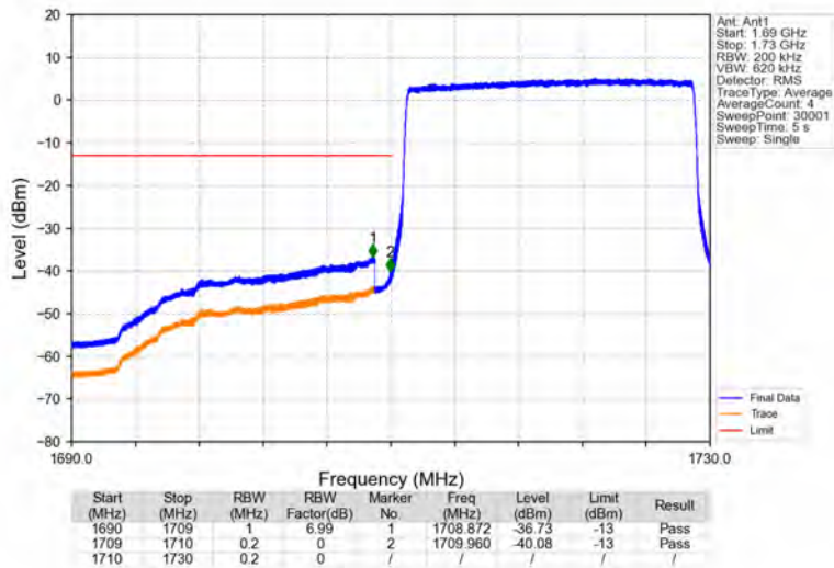
Band4_20MHz_QPSK_LCH_1720MHz_RB_100_0_NTNV
