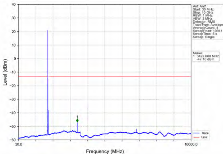
Band4_20MHz_16QAM_LCH_1720MHz_RB_1_0_NTNV
