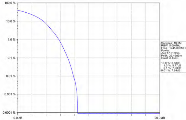
Band4_20MHz_QPSK_HCH_1745MHz_RB_100_0_NTNV
