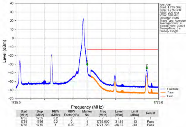
Band4_20MHz_QPSK_HCH_1745MHz_RB_1_99_NTNV
