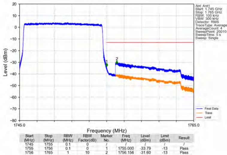
Band4_10MHz_QPSK_HCH_1750MHz_RB_50_0_NTNV
