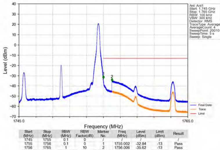
Band4_10MHz_QPSK_HCH_1750MHz_RB_1_49_NTNV
