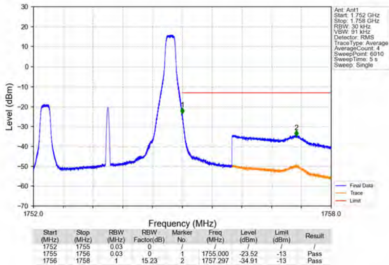
Band4_3MHz_QPSK_HCH_1753.5MHz_RB_1_14_NTNV
