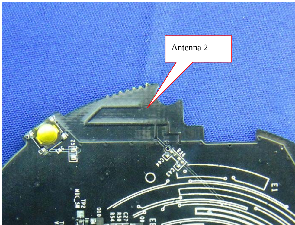
(19) EUT Photo
