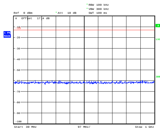
GSM 1900 CH-Middle 30MHz~1GHz
