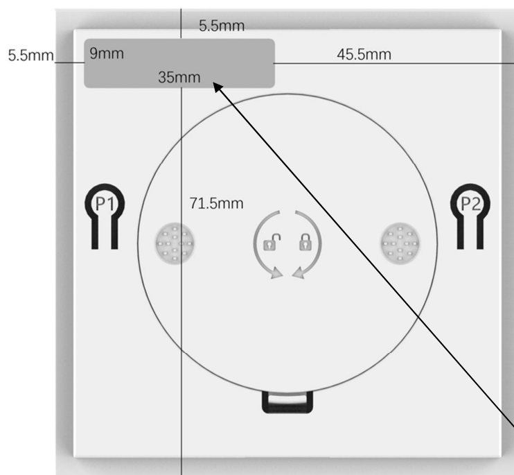
W5系列铭牌示意图
