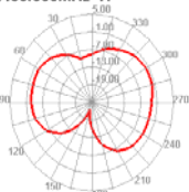
2450.000MHz H
