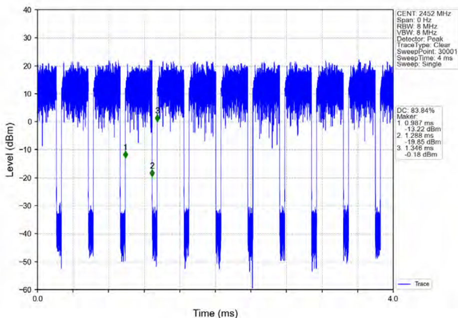
802.11ax(HE40)_HCH_2452MHz_RU484_Left_Ant1 (MIMO)_NTNV
