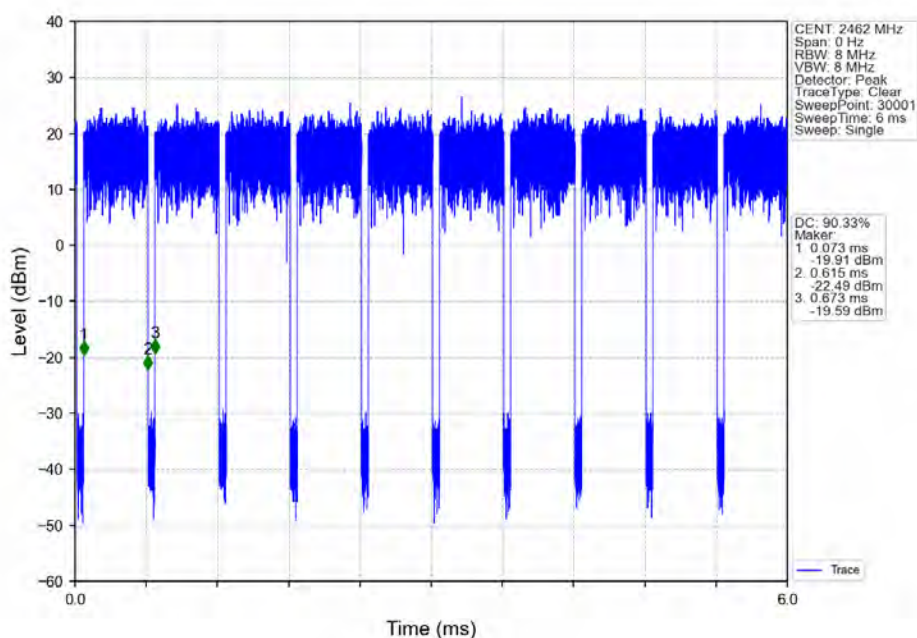
802.11ax(HE20)_HCH_2462MHz_RU242_Left_Ant2 (MIMO)_NTNV
