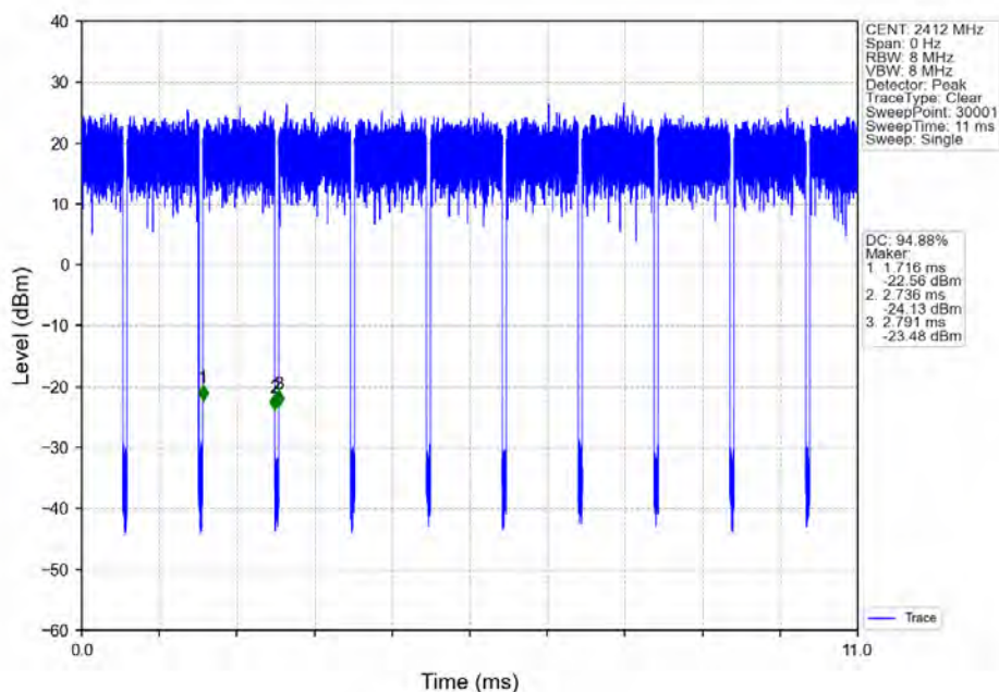
802.11ax(HE20) LCH_2412MHz_RU242_Left_Ant1 (MIMO) NTN
