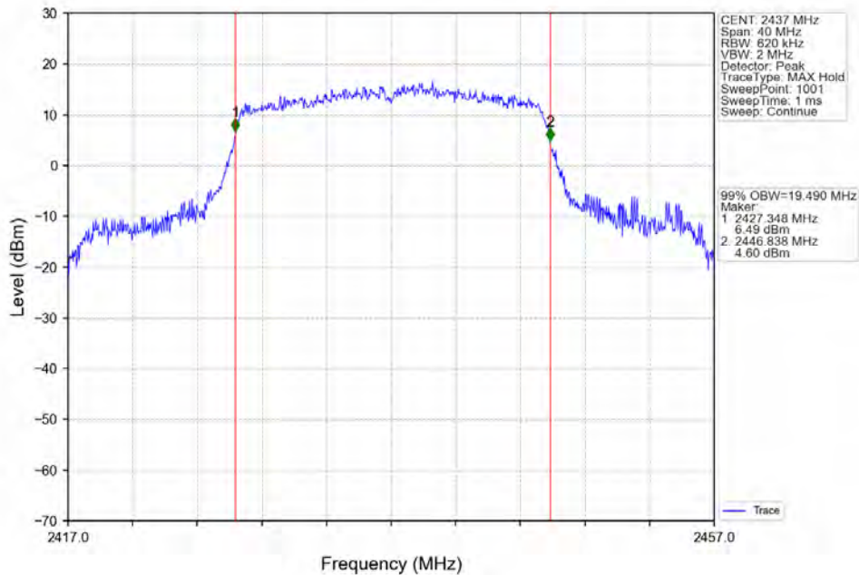
802.11ax(HE20)_MCH_2437MHz_RU242_Left_Ant1 (MIMO)_NTNV
