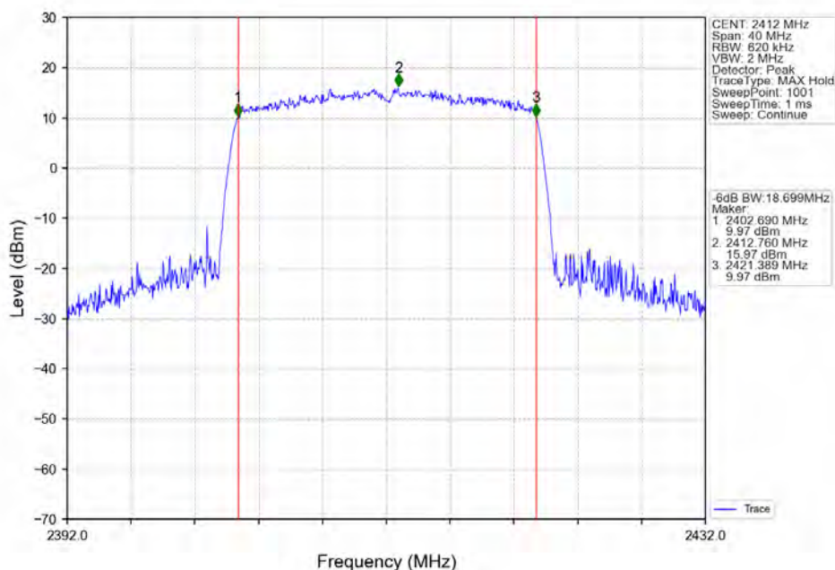
802.11ax(HE20) LCH_2412MHz_RU242_Left_Ant1 (MIMO) NTN
