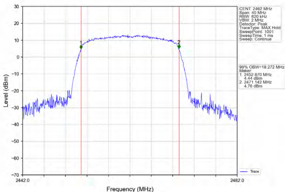
802.11ax(HE20)_HCH_2462MHz_RU242_Left_Ant1 (MIMO)_NTNV
