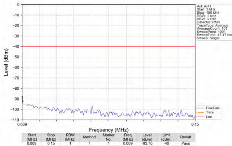
Band48_3550.2MHz_GMSK_SISO_Ant1_NTNV
