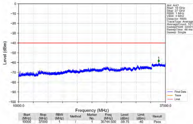
Band48_3625MHz_AWGN_SISO_Ant1_NTNV
