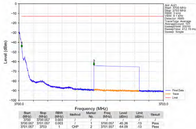
Band48 3699.8MHz_GMSK_SISO_Ant1_NTNV_AGC+3
