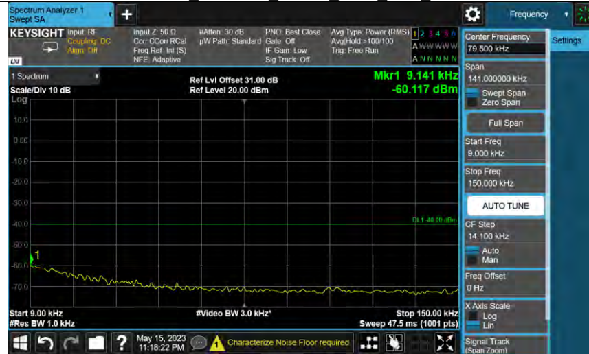
Band48_3625MHz_AWGN_SISO_Ant1_NTNV
