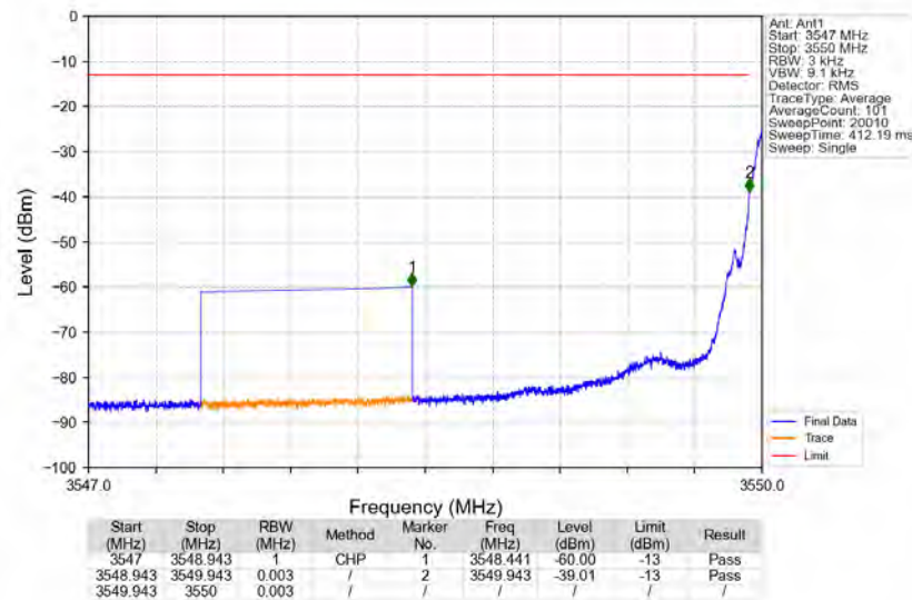
Band48 3550.2MHz_GMSK_SISO_Ant1_NTNV_AGC
