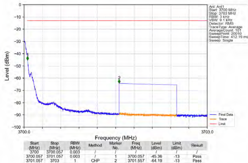
Band48 3699.8MHz_GMSK_SISO_Ant1_NTNV_AGC+3
