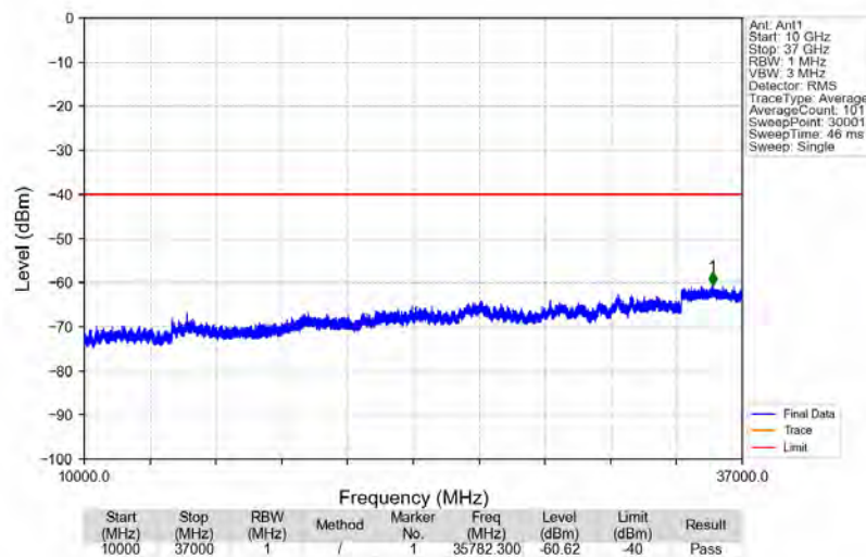
Band48_3625MHz_GMSK_SISO_Ant1_NTNV
