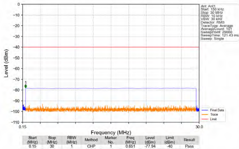
Band48_3550.2MHz_GMSK_SISO_Ant1_NTNV
