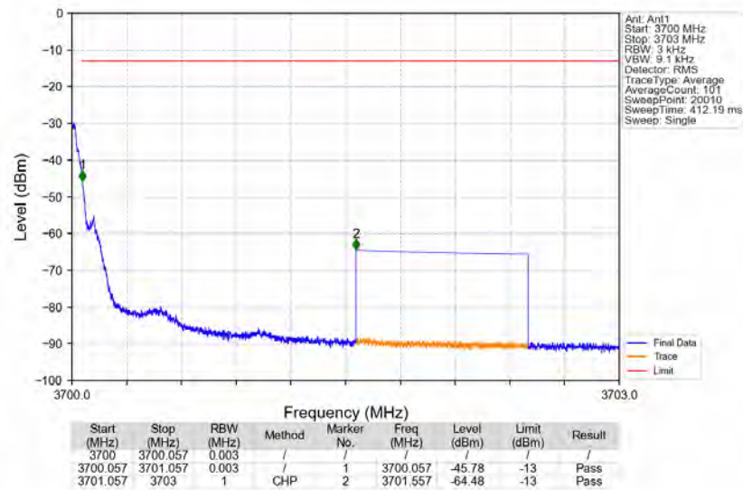
Band48 3699.8MHz_GMSK_SISO_Ant1_NTNV_AGC
