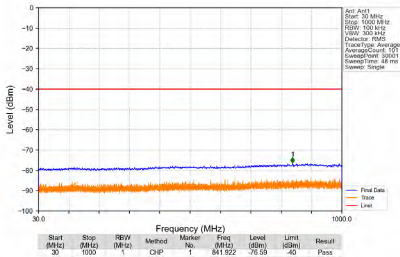
Band48_3625MHz_AWGN_SISO_Ant1_NTNV
