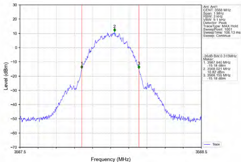
Band48_3568MHz_GMSK_SISO_Ant1_NTNV_Output_AGC+3
