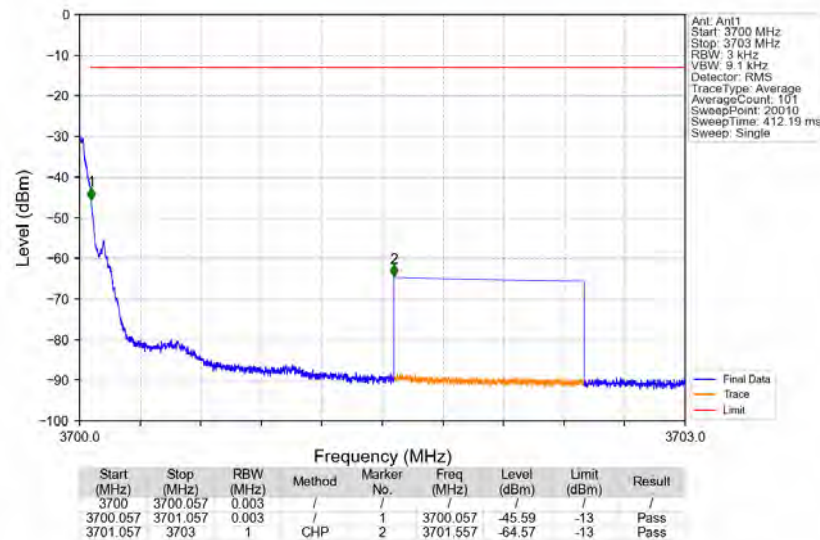
Band48 3699.8MHz_GMSK_SISO_Ant1_NTNV_AGC
