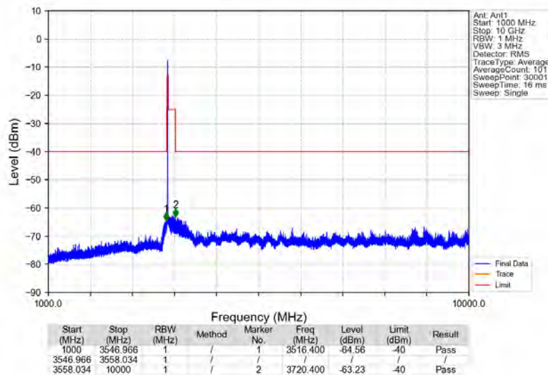
Band48_3552.5MHz_AWGN_SISO_Ant1_NTNV
