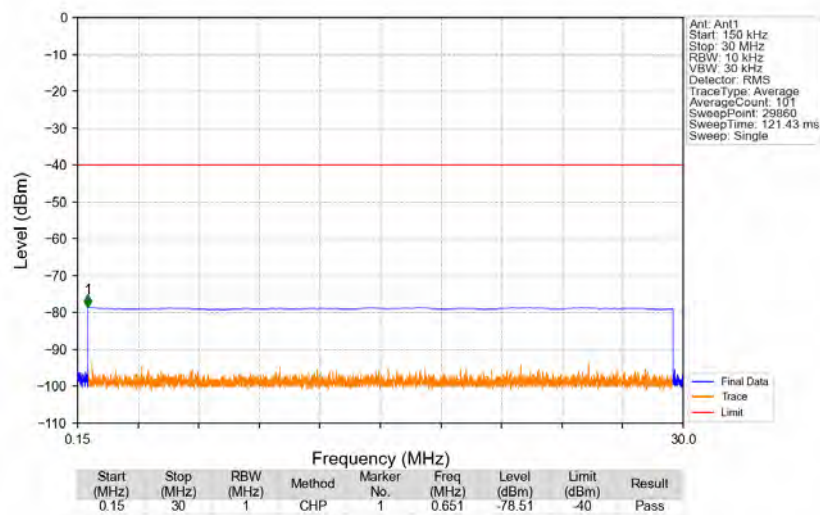
Band48_3625MHz_GMSK_SISO_Ant1_NTNV
