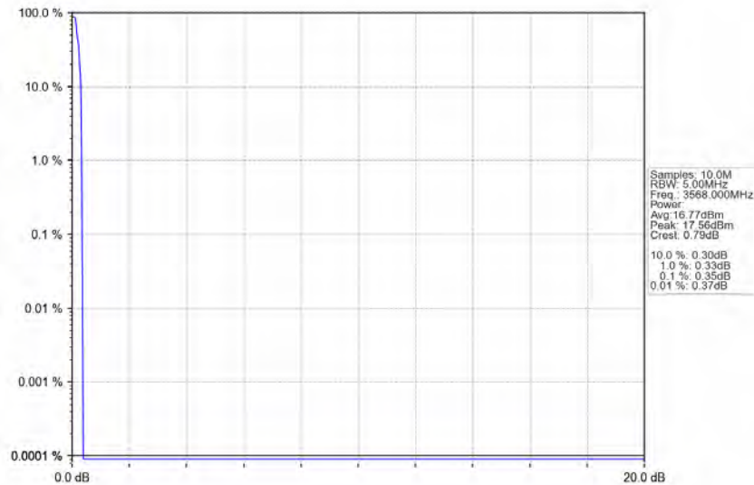
Band48_3568MHz_GMSK_SISO_Ant1_NTNV_AGC
