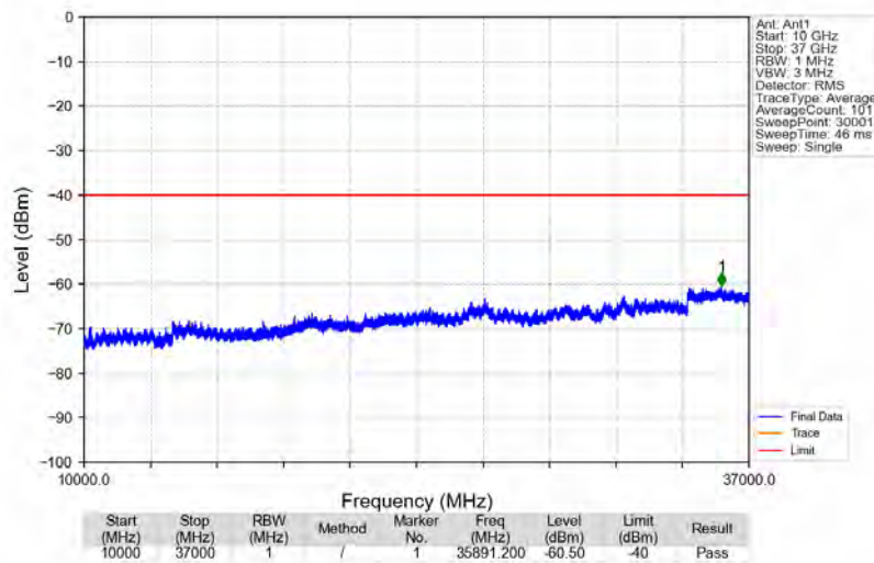
Band48 3699.8MHz_GMSK_SISO_Ant1_NTNV
