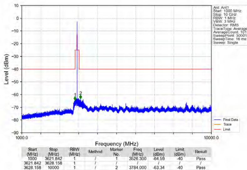
Band48_3625MHz_GMSK_SISO_Ant1_NTNV
