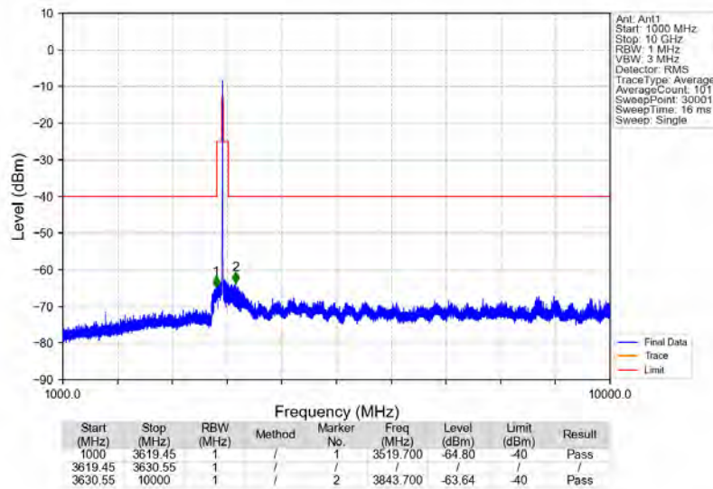
Band48_3625MHz_AWGN_SISO_Ant1_NTNV
