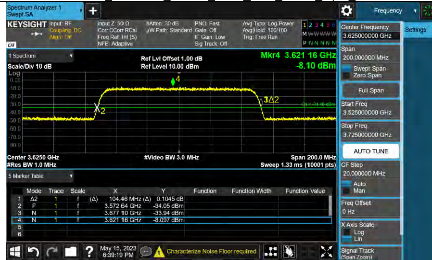
Band48 3625MHz AWGN SISO Ant1 NTN Input AGC+3
