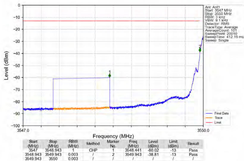
Band48 3550.2MHz_GMSK_SISO_Ant1_NTNV_AGC+3
