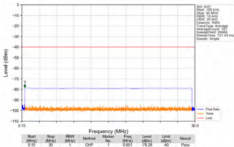
Band48_3625MHz_AWGN_SISO_Ant1_NTNV
