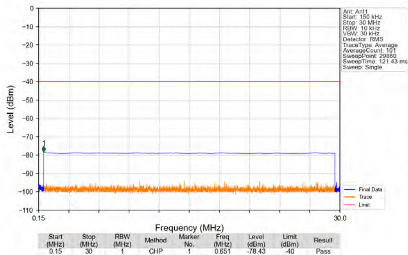
Band48_3699.8MHz_GMSK_SISO_Ant1_NTNV
