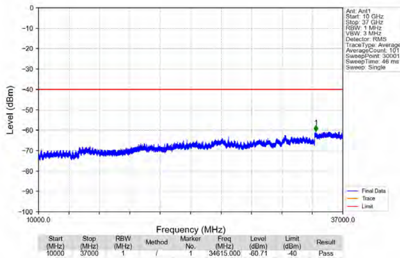
Band48 3550.2MHz_GMSK_SISO_Ant1_NTNV
