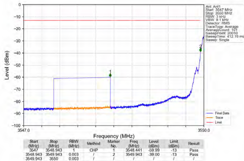
Band48 3550.2MHz_GMSK_SISO_Ant1_NTNV_AGC+3
