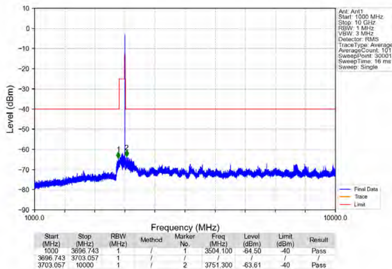
Band48 3699.8MHz_GMSK_SISO_Ant1_NTNV
