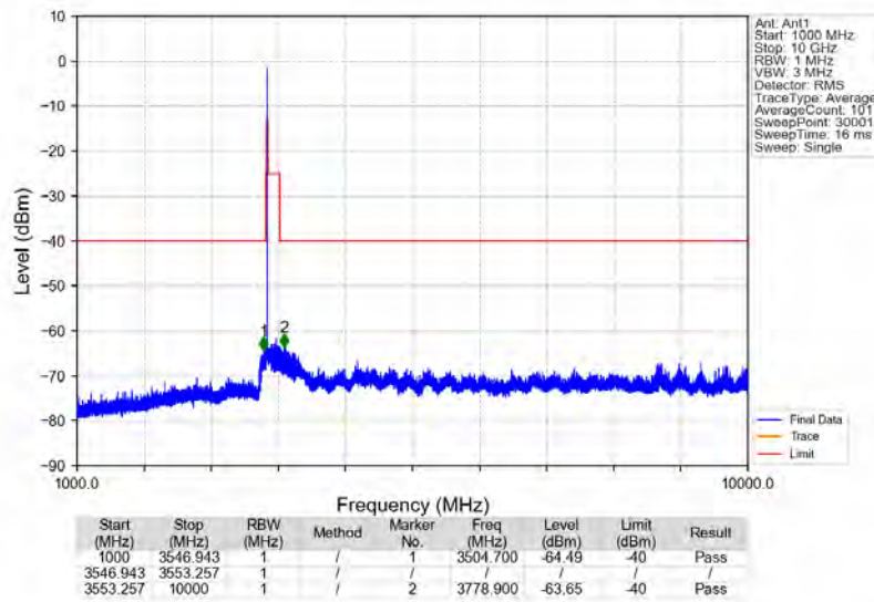
Band48 3550.2MHz_GMSK_SISO_Ant1_NTNV
