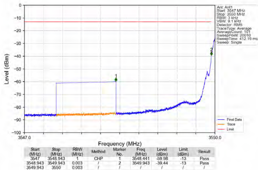
Band48 3550.2MHz_GMSK_SISO_Ant1_NTNV_AGC
