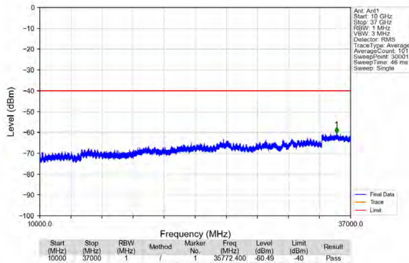
Band48_3552.5MHz_AWGN_SISO_Ant1_NTNV
