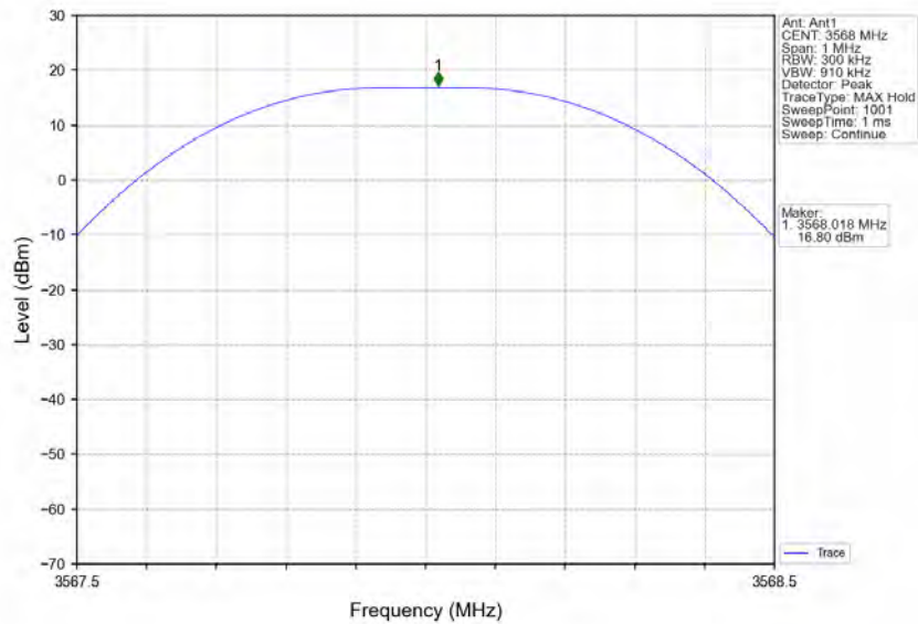
Band48_3568MHz_GMSK_SISO_Ant1_NTNV_AGC+3
