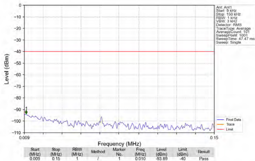
Band48_3625MHz_GMSK_SISO_Ant1_NTNV
