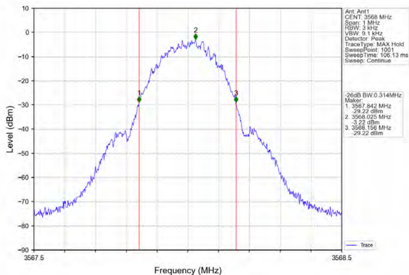
Band48_3568MHz_GMSK_SISO_Ant1_NTNV_Input_AGC+3
