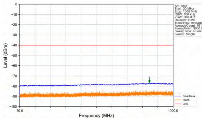
Band48_3625MHz_GMSK_SISO_Ant1_NTNV
