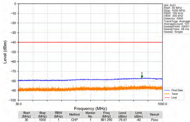
Band48_3699.8MHz_GMSK_SISO_Ant1_NTNV
