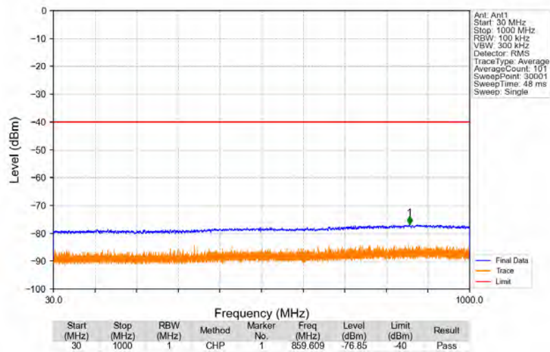
Band48_3550.2MHz_GMSK_SISO_Ant1_NTNV
