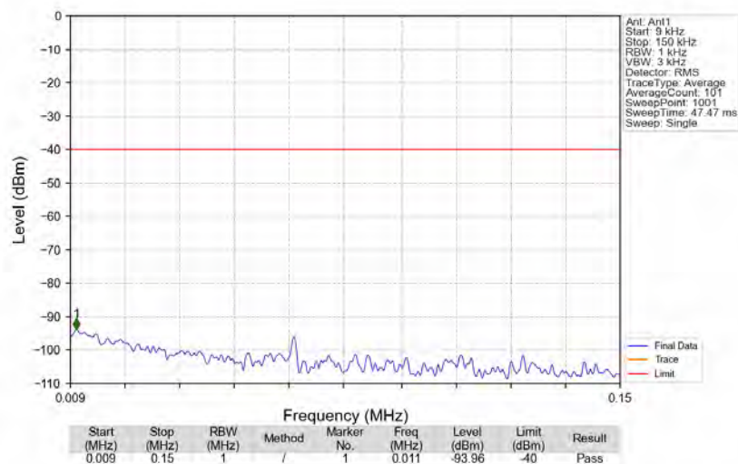
Band48_3699.8MHz_GMSK_SISO_Ant1_NTNV
