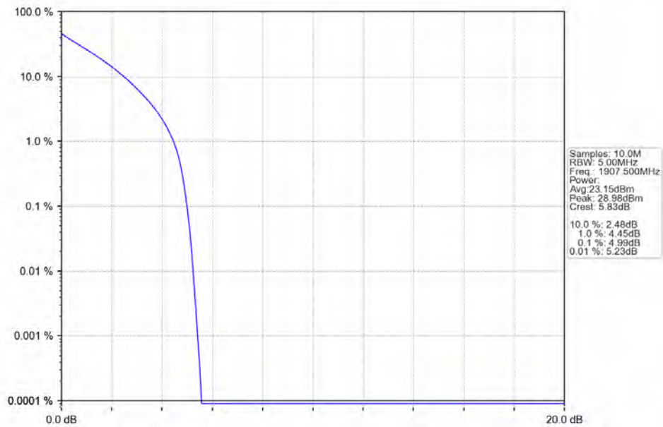
Band2 5MHz QPSK HCH 1907.5MHz RB 25 0 NTV
