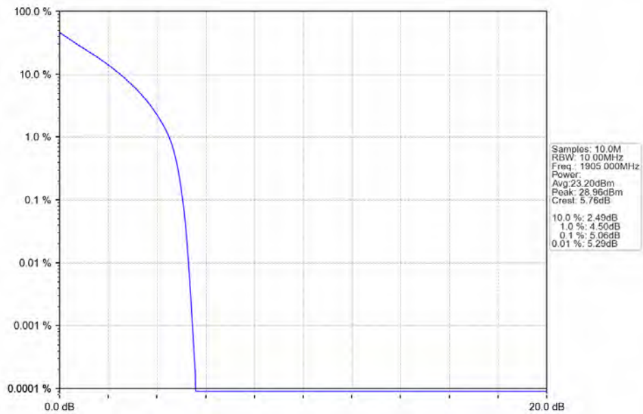
Band2 10MHz QPSK HCH 1905MHz RB 50 0 NTV
