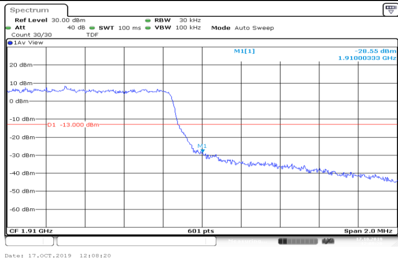
Band2-3MHz-QPSK-18615-15RB#0
