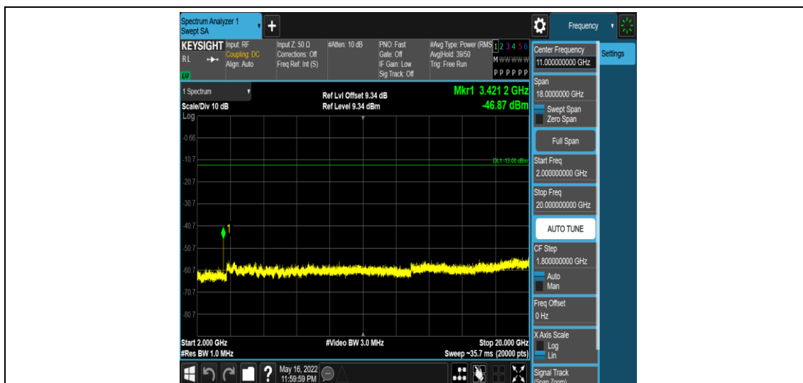
Band4-10MHz-QPSK-20000-1RB#0-Range5:2000~20000MHz
