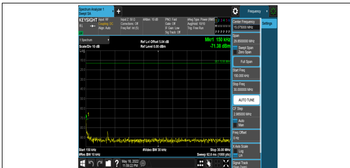
Band4-10MHz-QPSK-20000-1RB#0-Range2:0.15~30MHz
