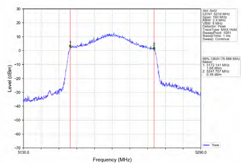
802.11ax(HEW80)_MCH_5210MHz_RU996_Left_Ant2_NTNV
