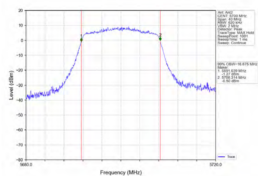
802.11a_HCH_5700MHz_Ant2_NTNV
