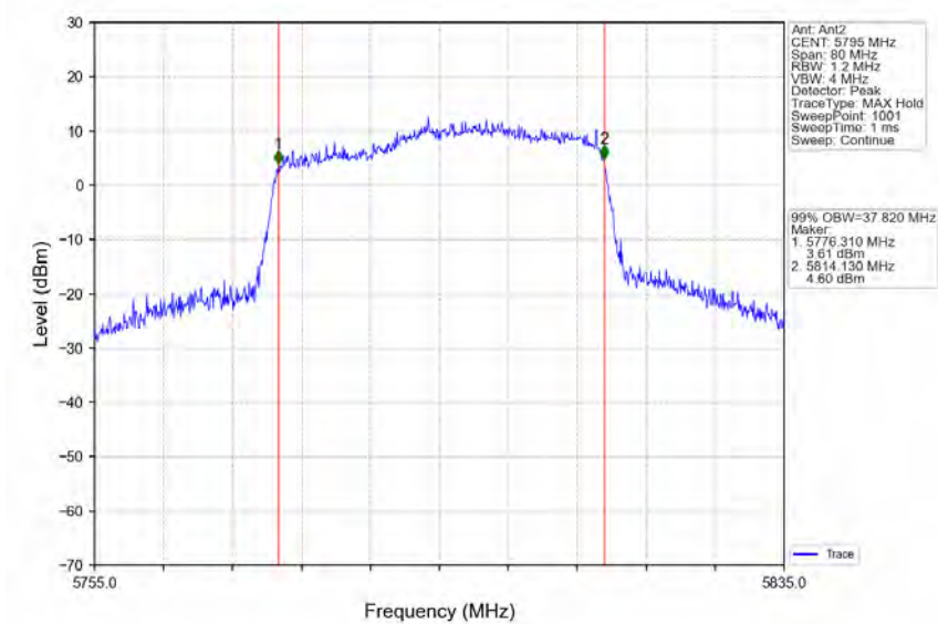
802.11ax(HEW40)_HCH_5795MHz_RU484_Left_Ant2_NTNV
