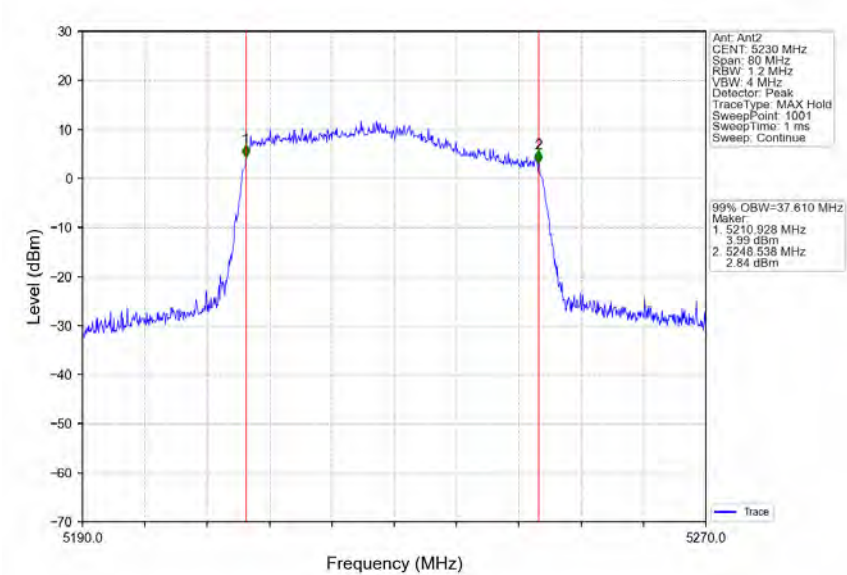
802.11ax(HEW40)_HCH_5230MHz_RU484_Left_Ant2_NTNV
