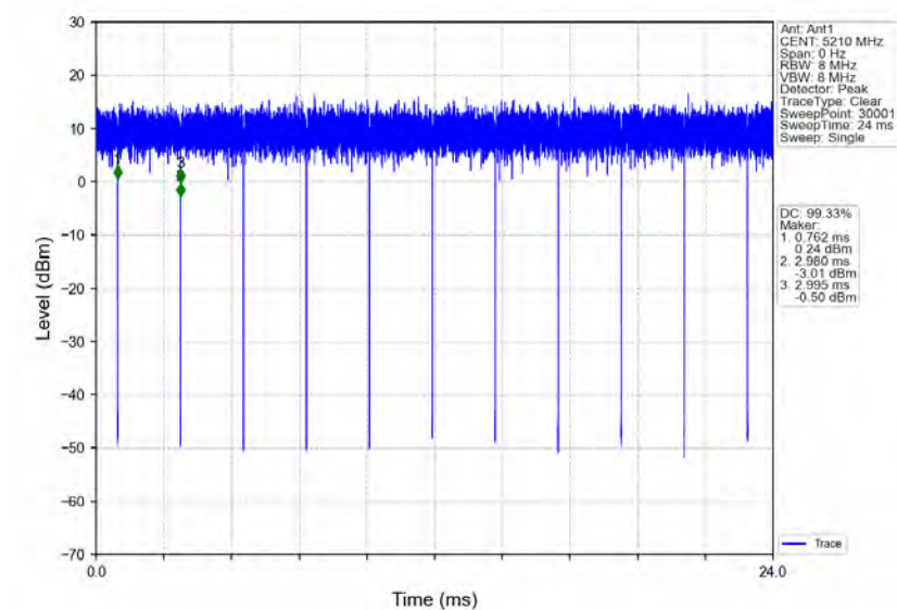
802.11ax(HEW80)_MCH_5210MHz_RU996_Left_Ant1_NTNV
