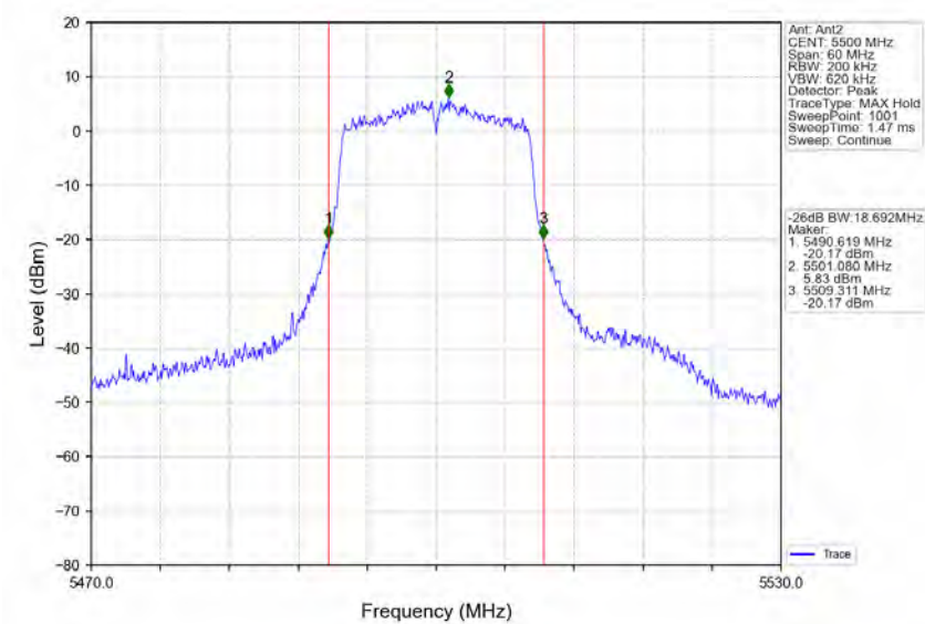
802.11a_LCH_5500MHz_Ant2_NTNV
