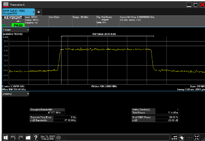
n41_50MHz_30kHz_2592.99MHz_CP-OFDM QPSK_RB133@0
