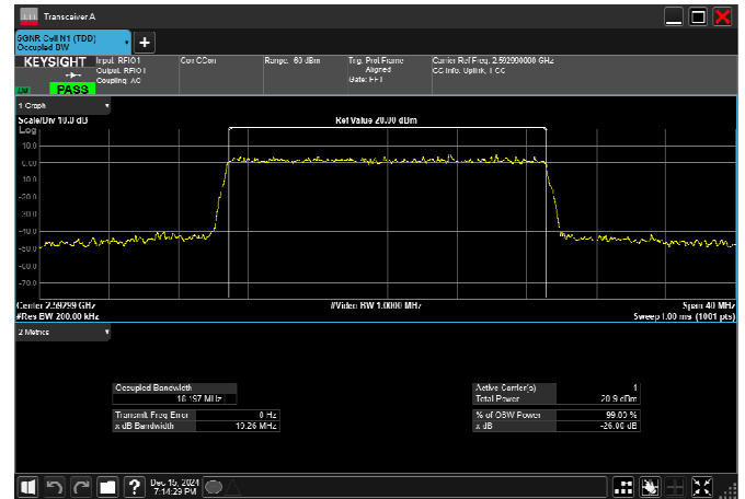
n41_30MHz_30kHz_2592.99MHz_DFT-s-OFDM \pi/2 BPSK_RB75@0
