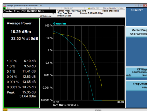
B12-3M-Mid CH-PAPR-Q16
