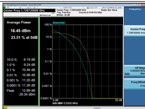
B4-10M-Mid CH-PAPR-Q16
