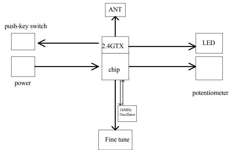
ABE2402X1- 66804TXV1-block diagram
