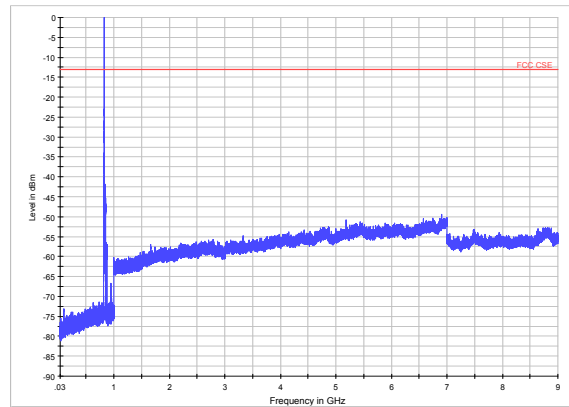
WCDMA Band V CH-Low 30MHz ~ 9GHz
