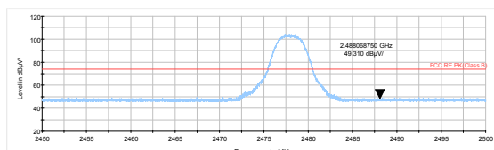
BT UHD 2M \pi/4 -DQPSK 2478MHz: Peak
