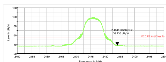
BT UHD 4M \pi/4 -DQPSK 2476MHz: Average
