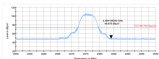
BT UHD 4M \pi/4 -DQPSK 2476MHz: Peak
