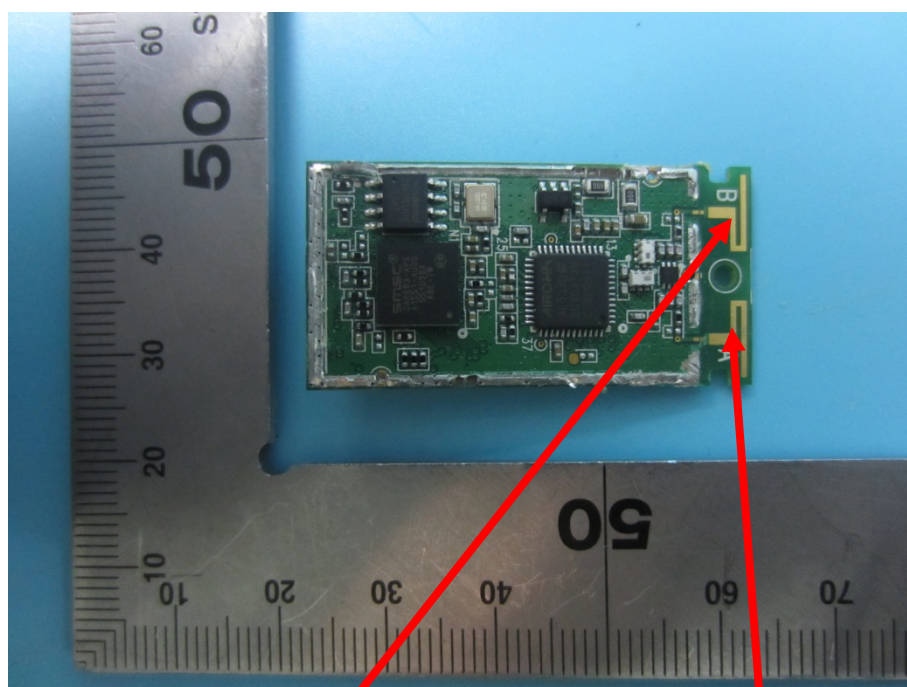
Antenna A
