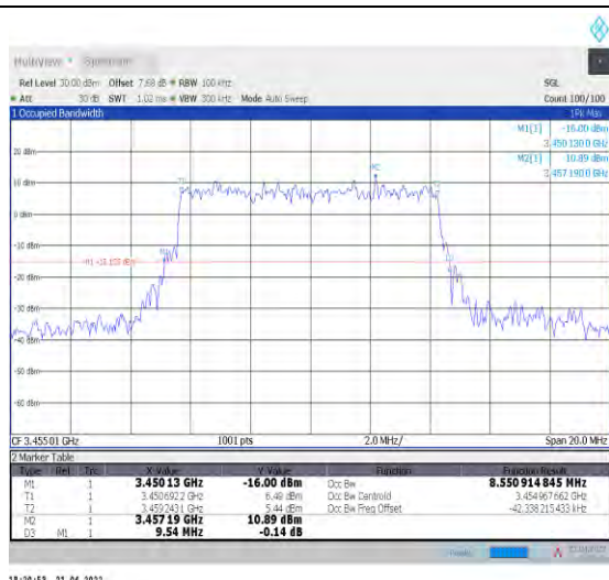
1-N78-3450-3550--30-10-L-5-DFT-256QAM-Outer_Full -24@0-Ant1-8.551-9.540-≤10-PASS
