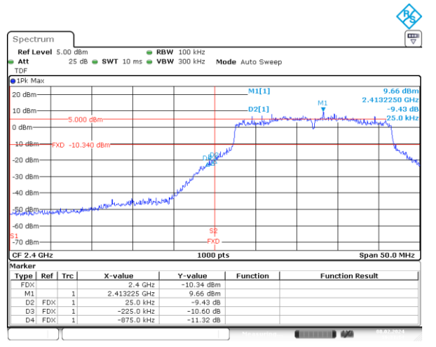
BE-NR, SISO-A, 802.11ax40-HE0, Ch3
