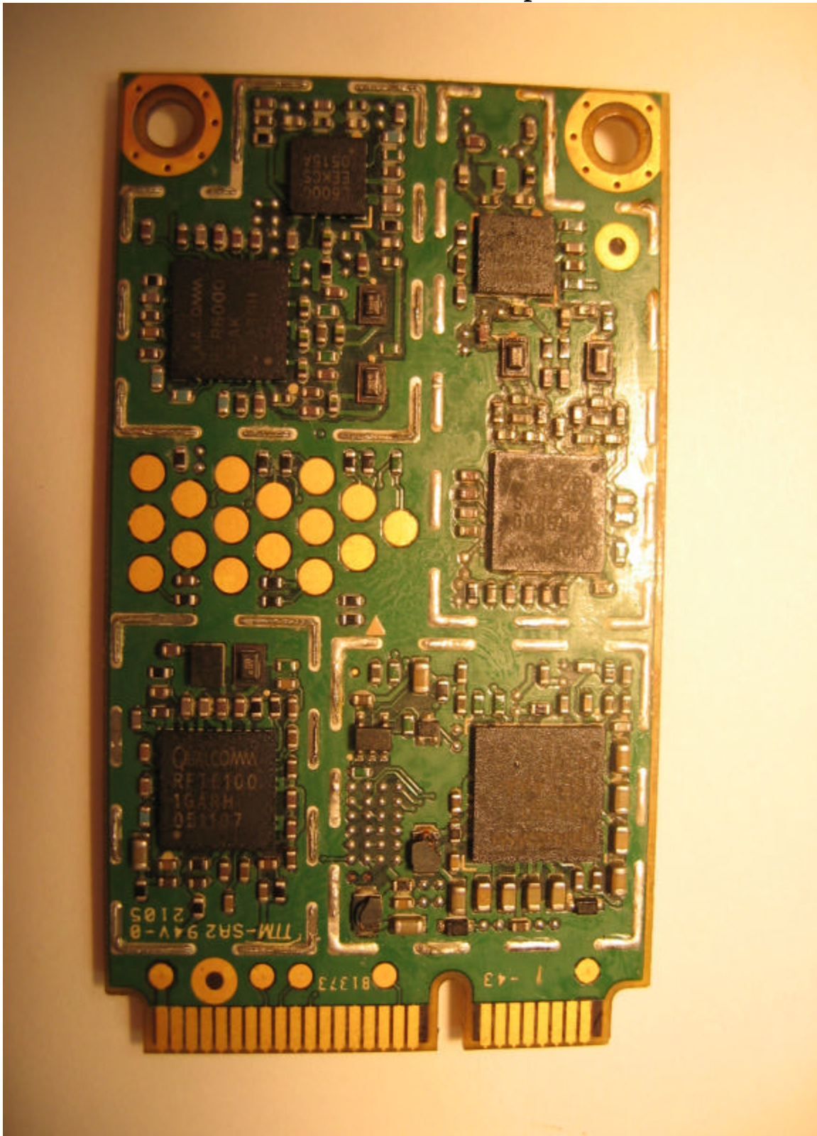
Bottom Side Without Shields Mini Express Card
