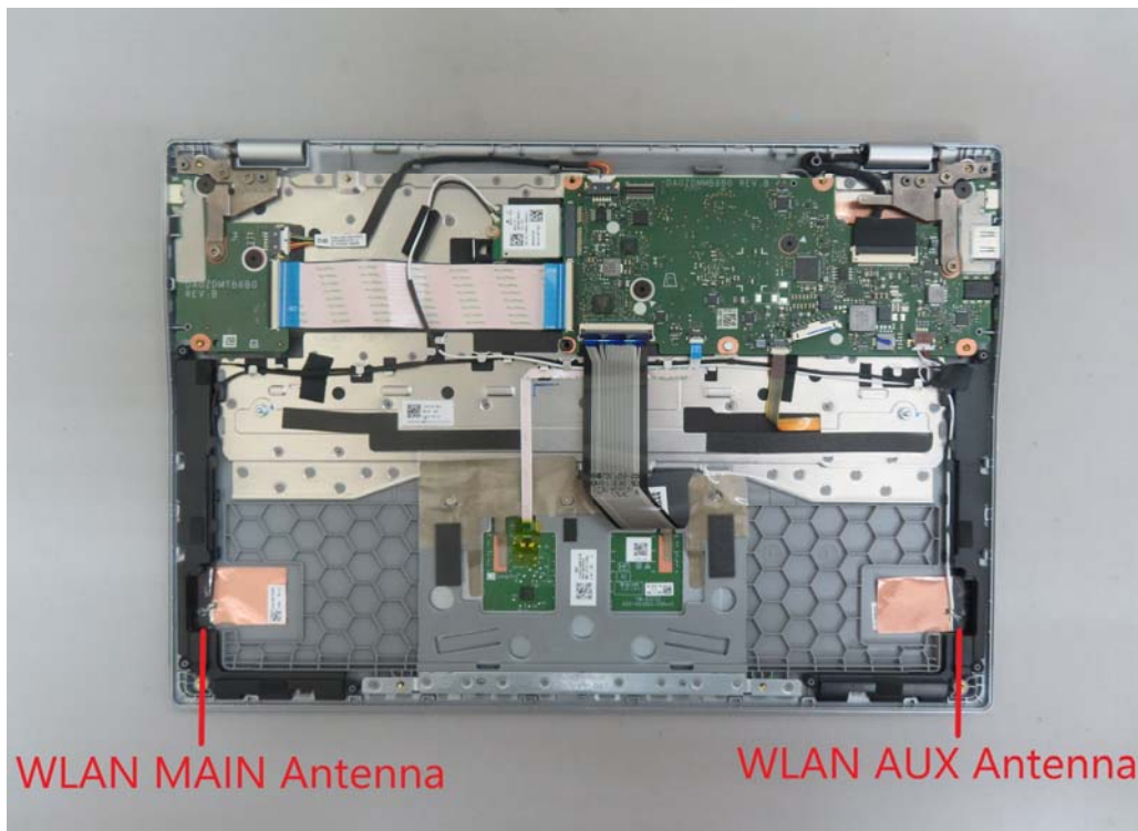
Antenna
