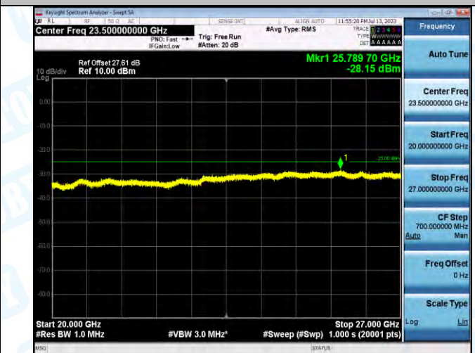
Band7_Band7_20MHz_QPSK_20850_1RB#0_20000~27000_20000~27000
