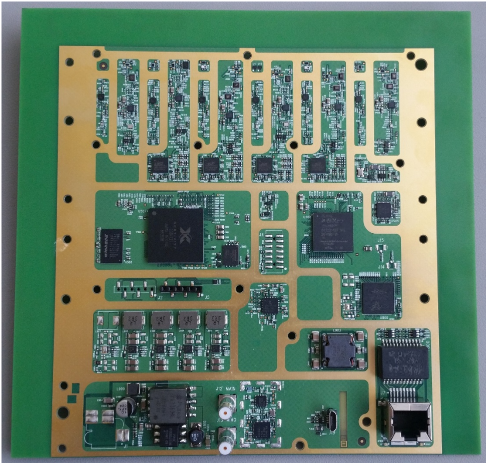
PCB Side_2_no shield – CU
