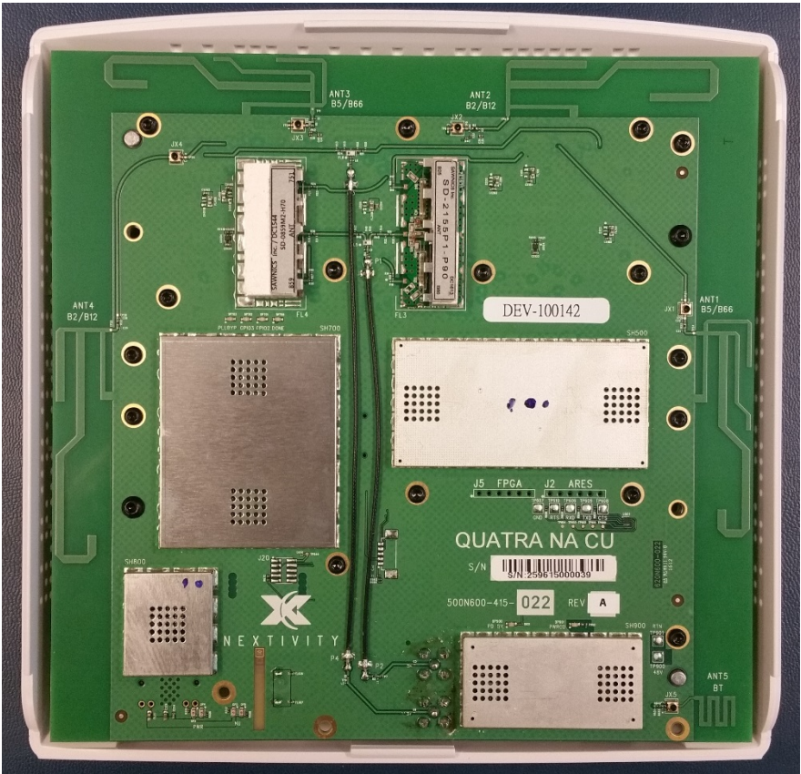
PCB Side_1 - CU
