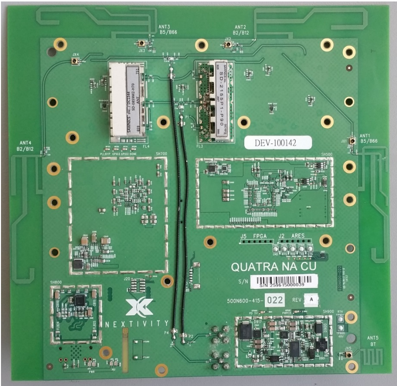
PCB Side_1_no shield - CU
