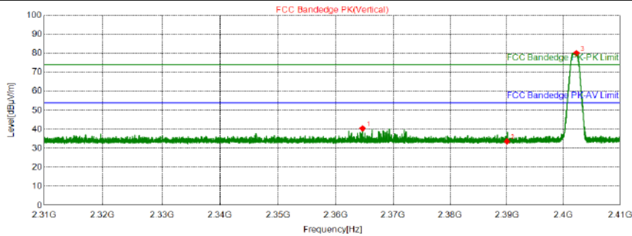
BLE_1M_2402_Ant1/ Vertical
