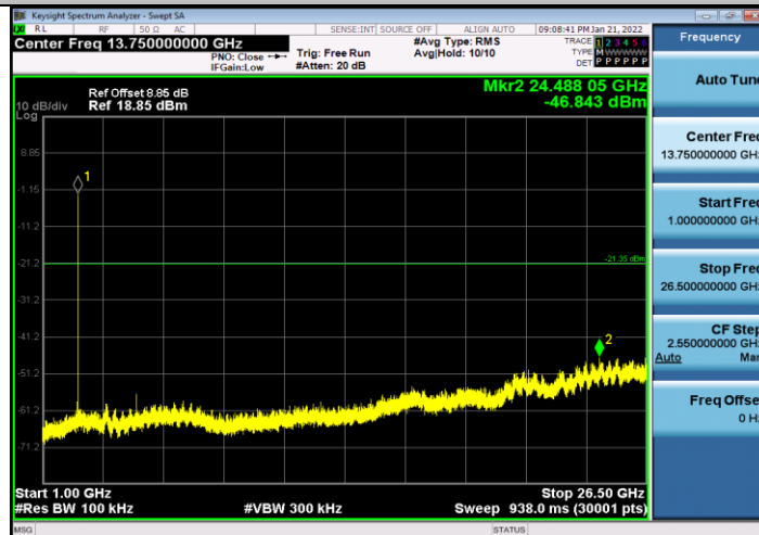
BLE_1M_Ant1_2480_1000~26500
