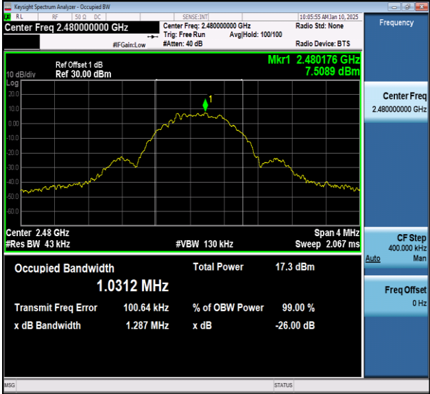
BLE_500K-Ant1-2480
