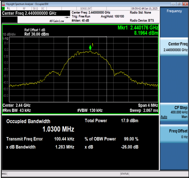
BLE_500K-Ant1-2440
