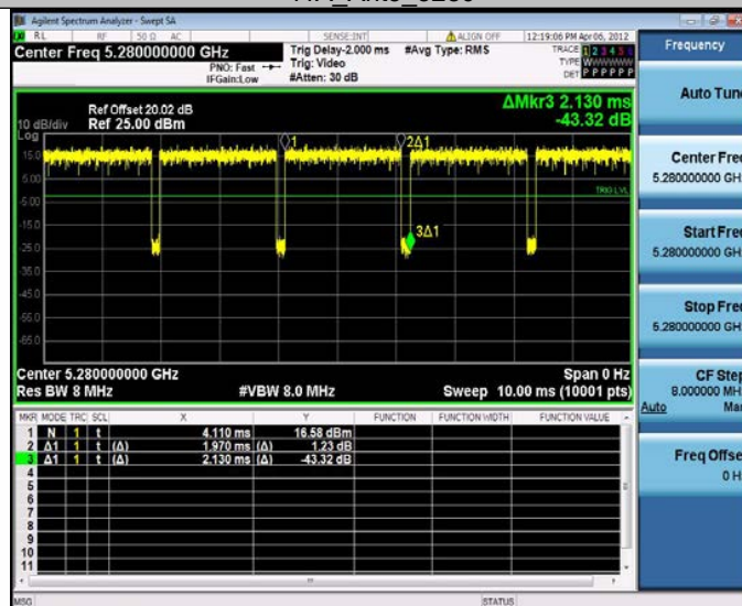
11A_Ant3_5280
