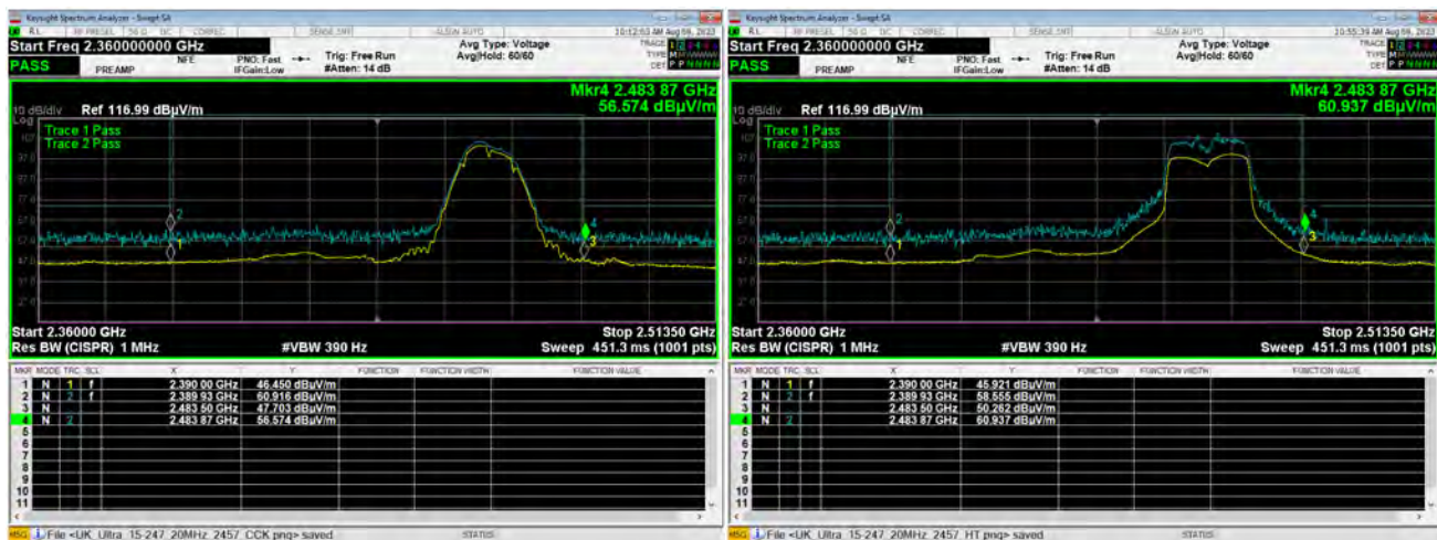
CCK_2462
