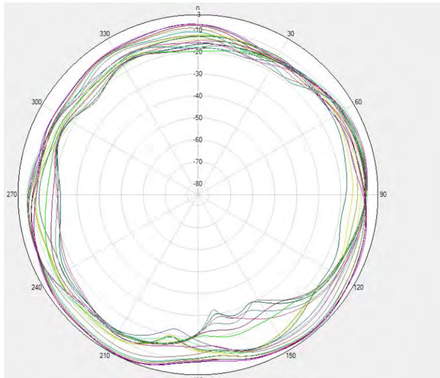
Flip- LTEB38/41&N38/N41 MIMO1 \Phi=90^\circ
