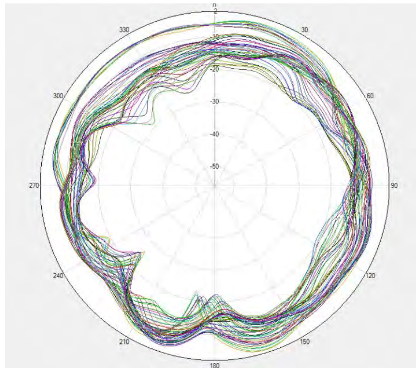
Unflip- N77/N78 MIMO1 \Phi=90\text{deg}
