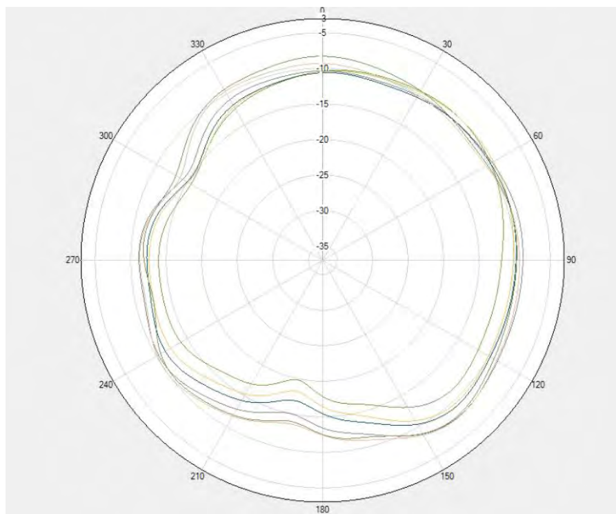
Unflip- LTE B40&N40 MIMO2 \Theta=90\text{deg}
