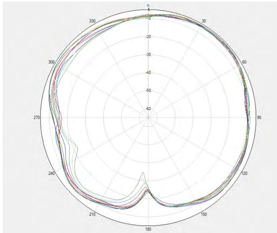
Flip- LTEB38/41&N38/N41MIMO2 \Phi=90\text{deg}
