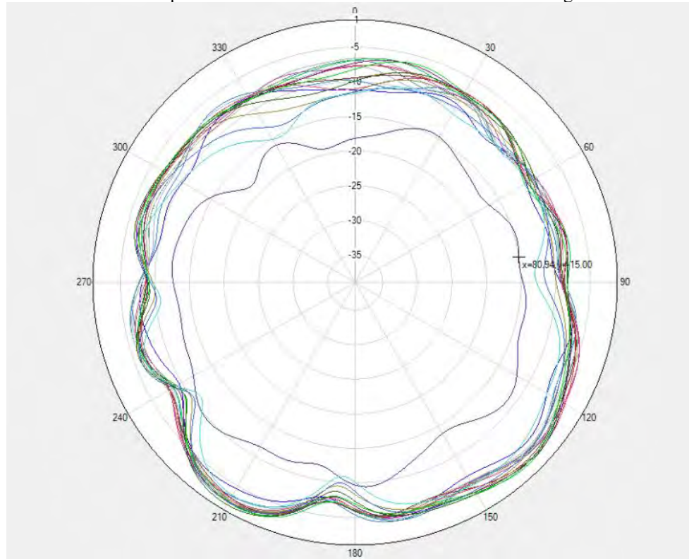
Unflip-WCDMA B1&LTE B1&NR N1 PRX Phi=90deg
