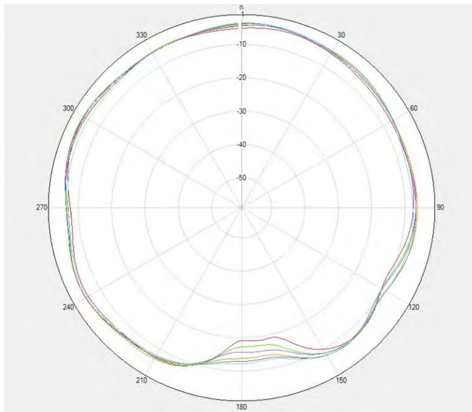
Unflip-LTE B40&N40 PRX \Theta=90\text{deg}
