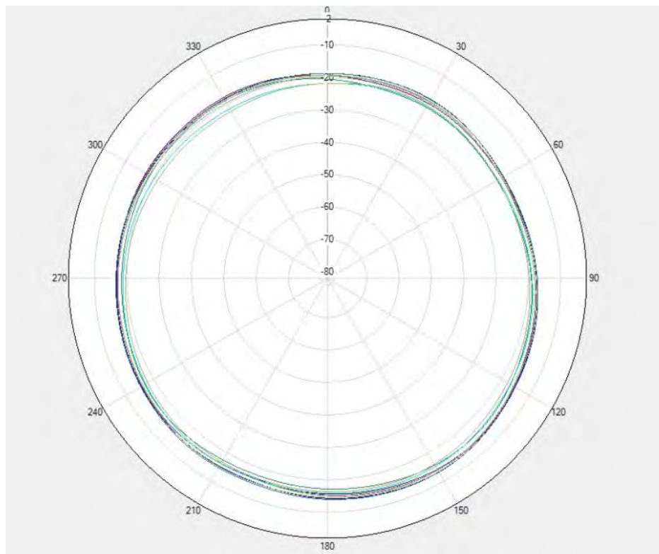
ENDC Flip LTE B5&NR N5 PRX \Theta=90\text{deg}
