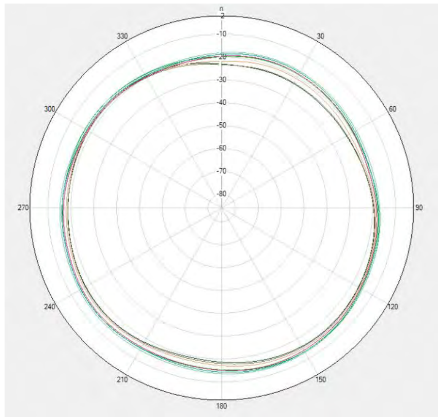
END C Flip LTE B8&NR N8 PRX Theta=90deg
