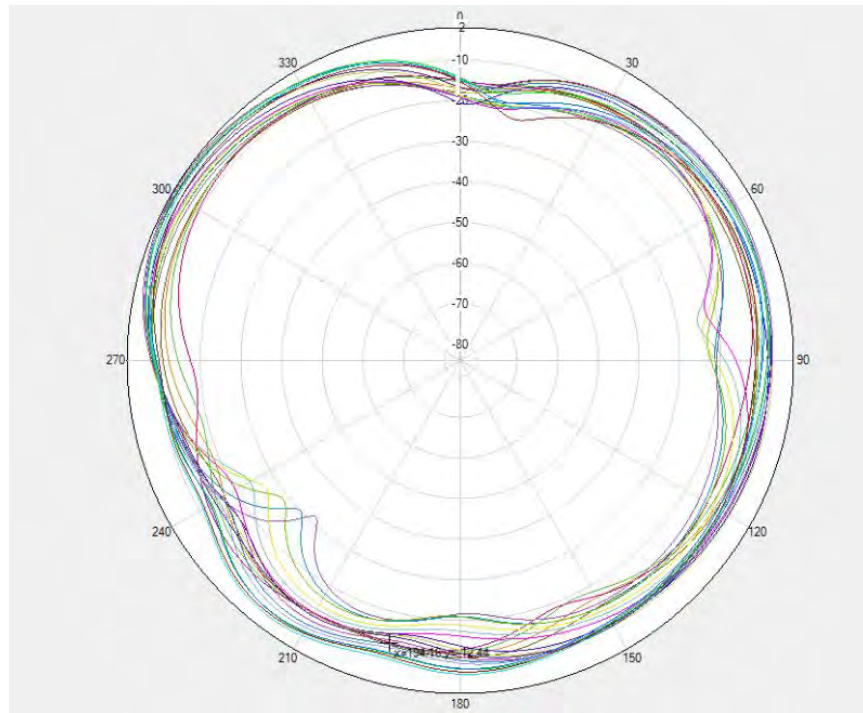
Flip- LTEB38/41&N38/N41 MIMO1 Theta=90deg
