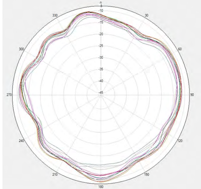
Unflip- GSM 850&WCDMA B5&LTE B5/B20& NR N5/N20 PRX Phi=90deg
