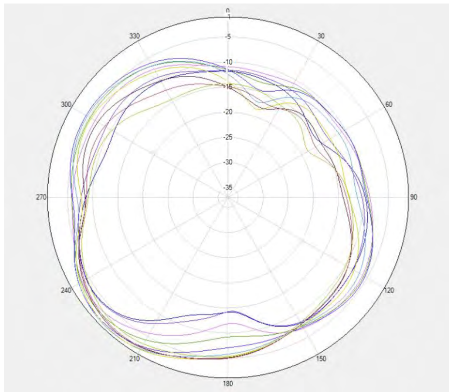
Flip- LTEB38/41&N38/N41 DRX Theta=90deg
