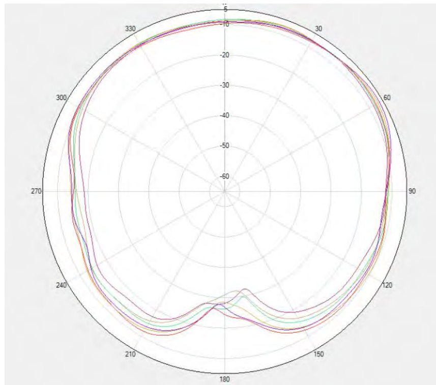
Flip- LTE B40&N40 MIMO2 \Phi=90\text{deg}
