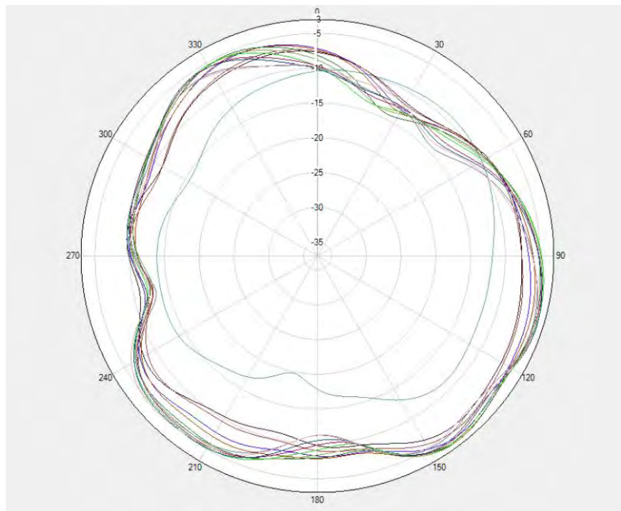
Unflip- LTEB38/41&N38/N41 MIMO2 \Theta=90^\circ
