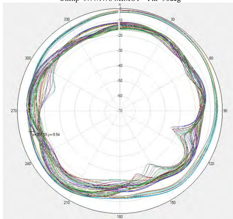
Flip- N77/N78 MIMO1 \Theta=90\text{deg}
