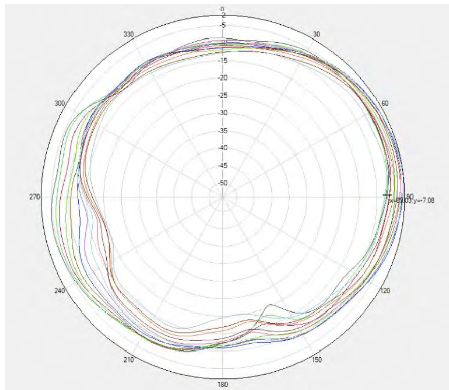
Flip-WCDMA B1&LTE B1&NR N1 PRX \Phi=90\text{deg}
