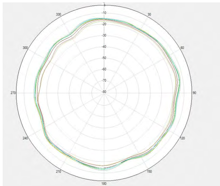
END C Flip LTE B8&NR N8 PRX Phi=0deg
