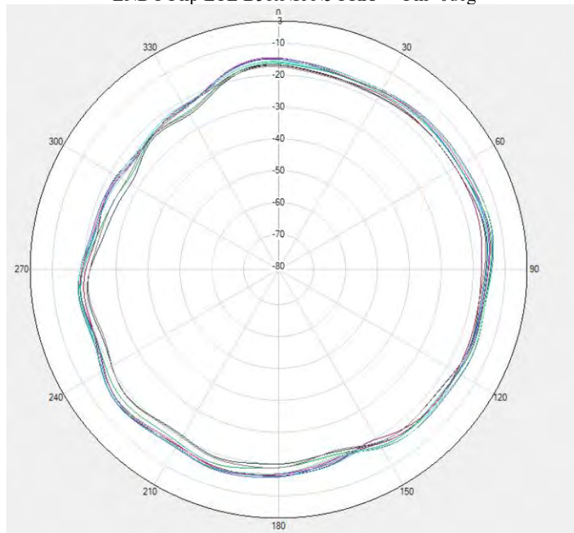
ENDC Flip LTE B5&NR N5 PRX Phi=90deg
