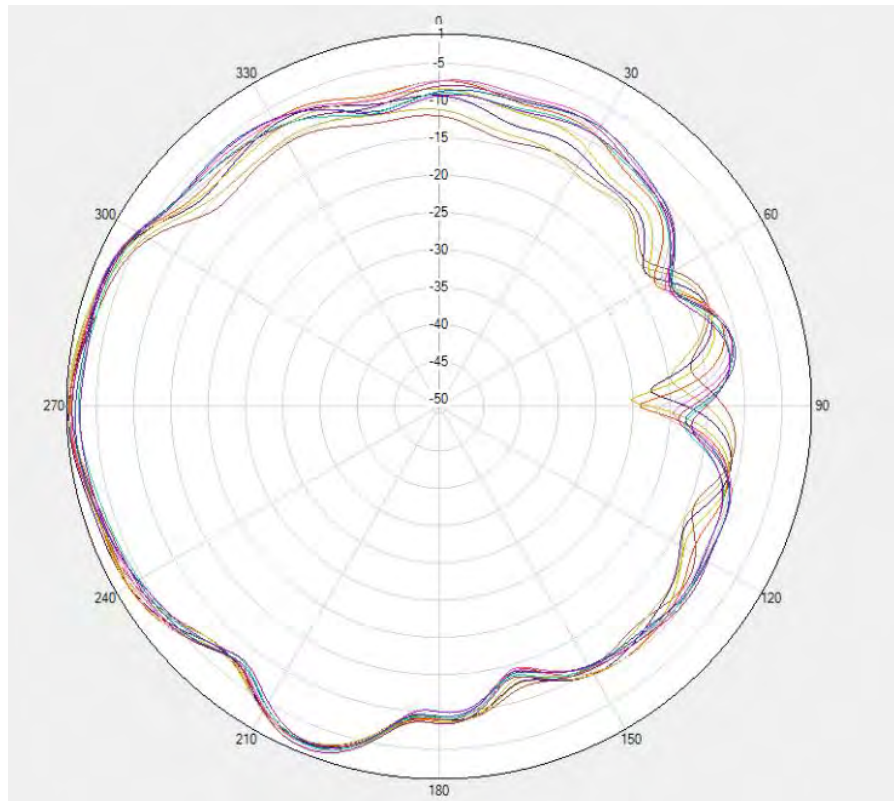
Unflip- LTE B7/38/41&N7/N38/N41 PRX Phi=0deg
