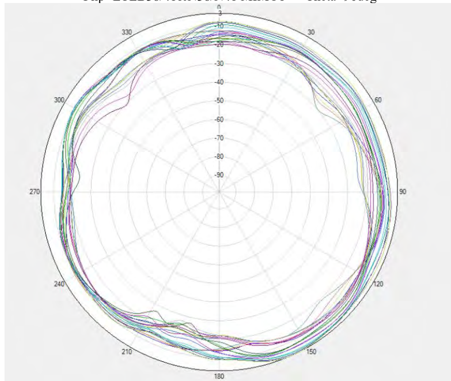
Flip- LTEB38/41&N38/N41 MIMO1 Phi=0deg
