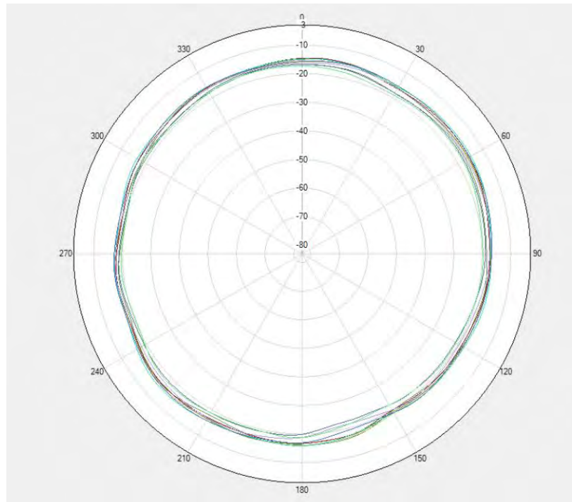
ENDC Flip LTE B5&NR N5 PRX Phi=0deg
