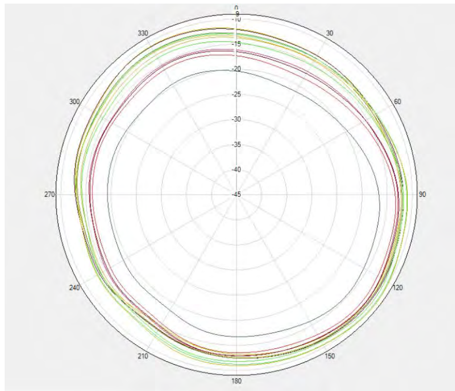
Flip- LTE B28&N28 Theta=90deg
