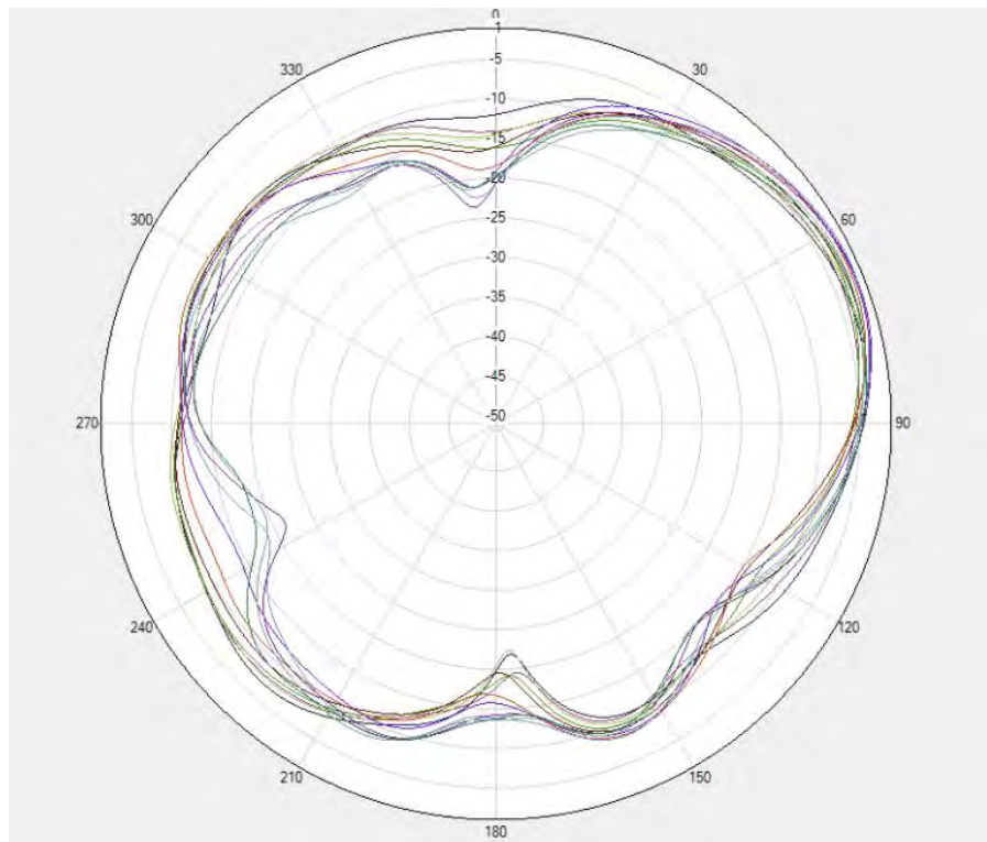
Flip- LTE B7/38/41&N7/N38/N41 PRX \Phi=90\text{deg}
