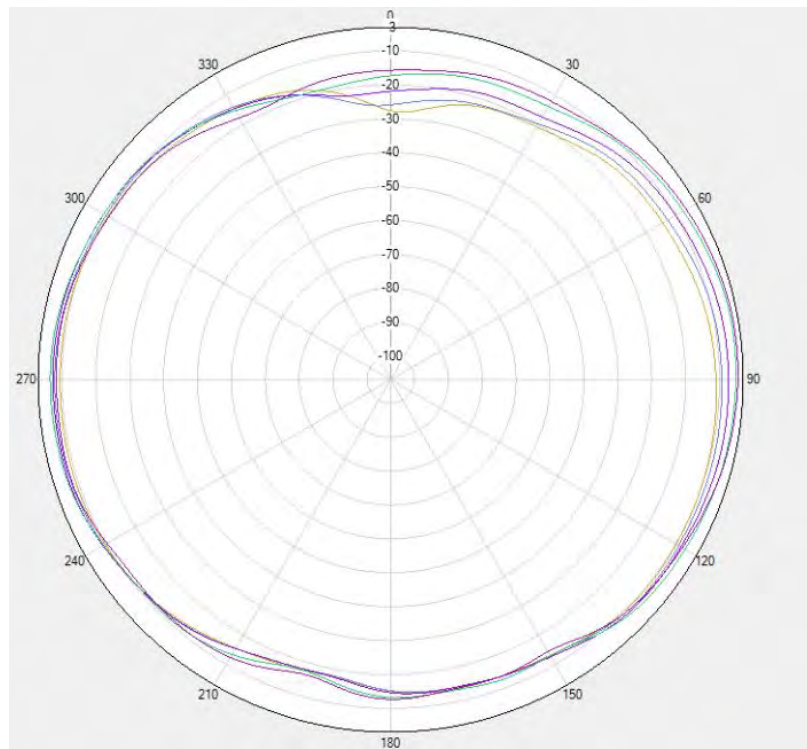
ENDC Flip LTE3/B4/B66 PRX \Phi=90\text{deg}
