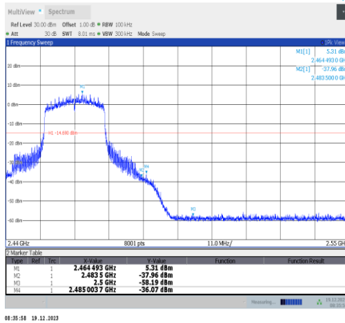
11ax20MIMO-Ant4-2462-PASS
