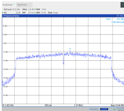
11ax20MIMO-Ant4-2462-PASS
