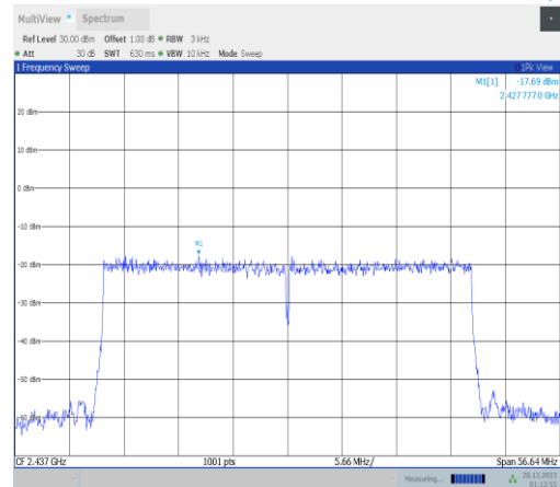
11ax40MIMO-Ant1-2437-PASS
