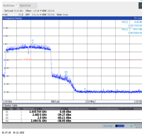
11ax40MIMO-Ant4-2452-PASS
