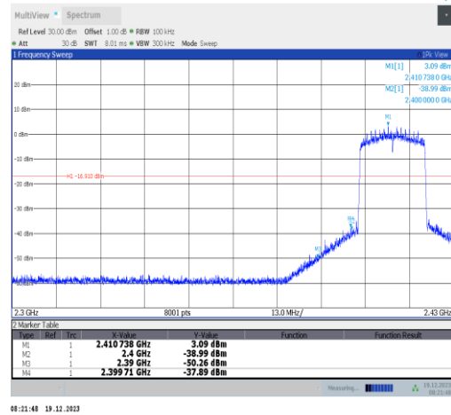
11ax20MIMO-Ant3-2412-PASS
