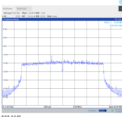
11ax20MIMO-Ant4-2437-PASS
