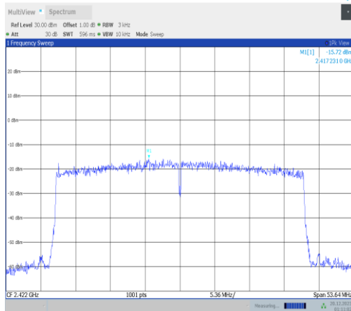
11ax40MIMO-Ant4-2422-PASS
