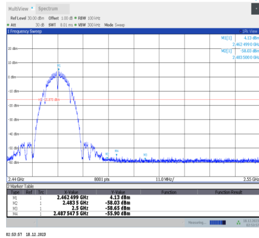
11b-Ant2-2462-PASS
