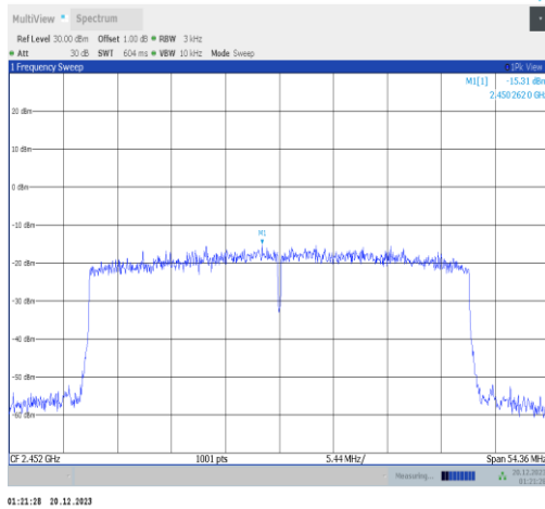
11ax40MIMO-Ant4-2452-PASS
