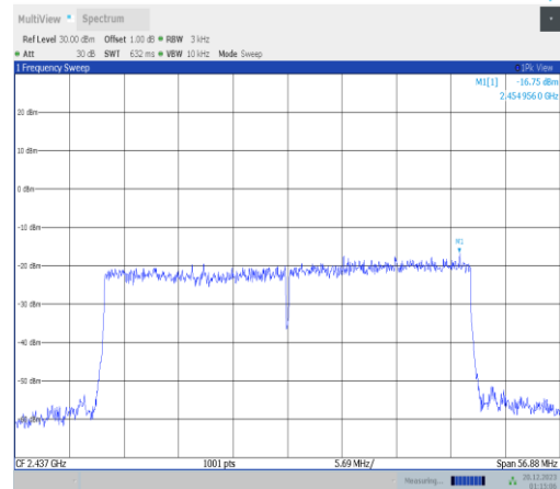
11ax40MIMO-Ant3-2437-PASS
