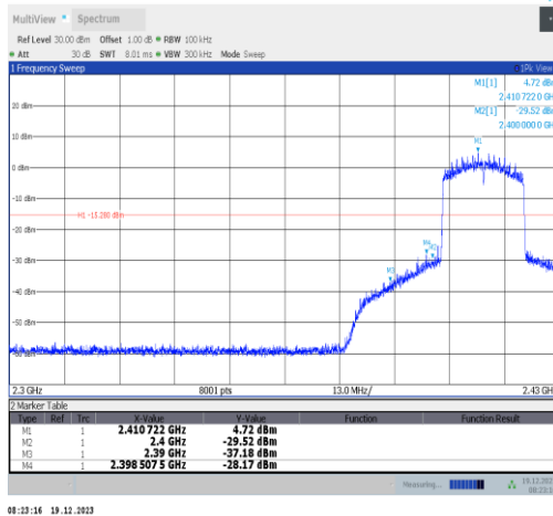
11ax20MIMO-Ant4-2412-PASS
