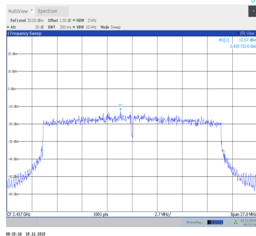
11ax20MIMO-Ant1-2437-PASS
