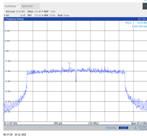
11ax20MIMO-Ant3-2437-PASS
