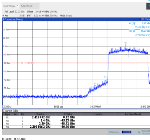
11ax40MIMO-Ant4-2422-PASS
