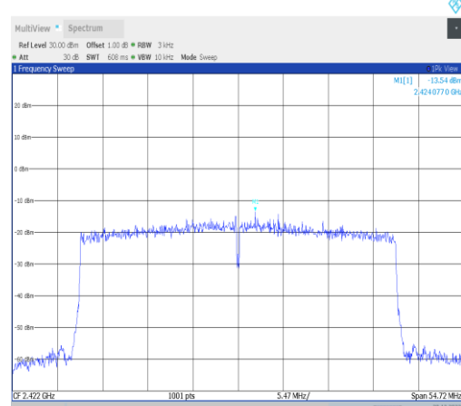
11ax40MIMO-Ant3-2422-PASS
