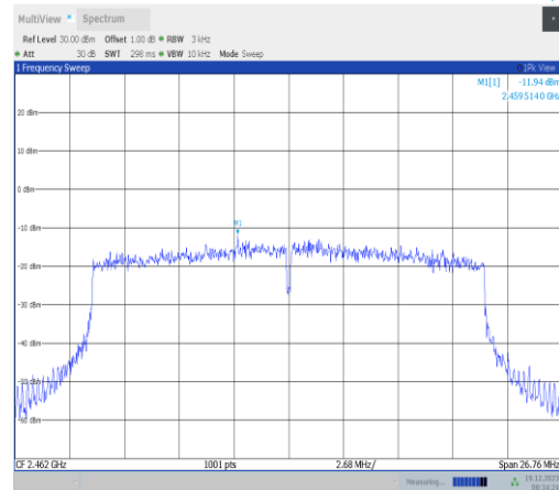
11ax20MIMO-Ant3-2462-PASS
