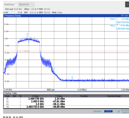
11ax20MIMO-Ant3-2462-PASS
