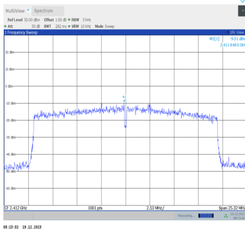
11ax20MIMO-Ant4-2412-PASS
