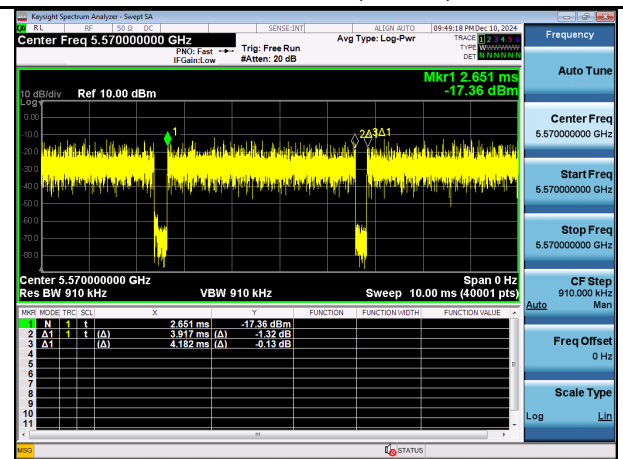
IEEE 802.11ax(HE160)
