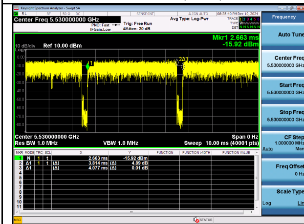
IEEE 802.11ax(HE80)
