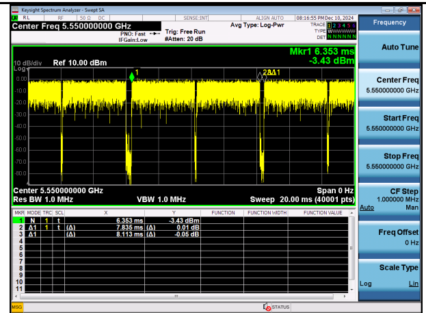
IEEE 802.11ac(VHT40)
