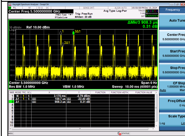
IEEE 802.11a
