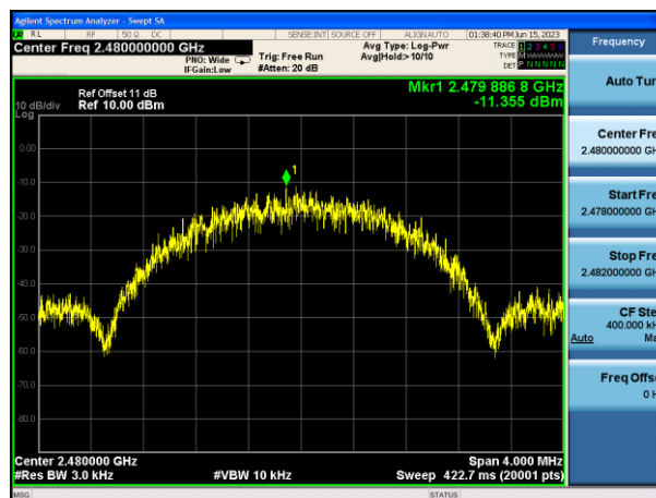
CH78 (2480MHz)
