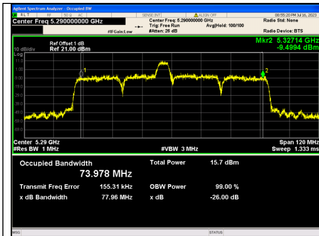
IEEE 802.11ax_Channel 58_80MHz_Antenna 0_RU&amp;Index 52RU44
