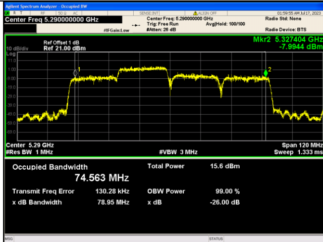
IEEE 802.11ax_Channel 58_80MHz_Antenna 0_RU&amp;Index 242RU62
