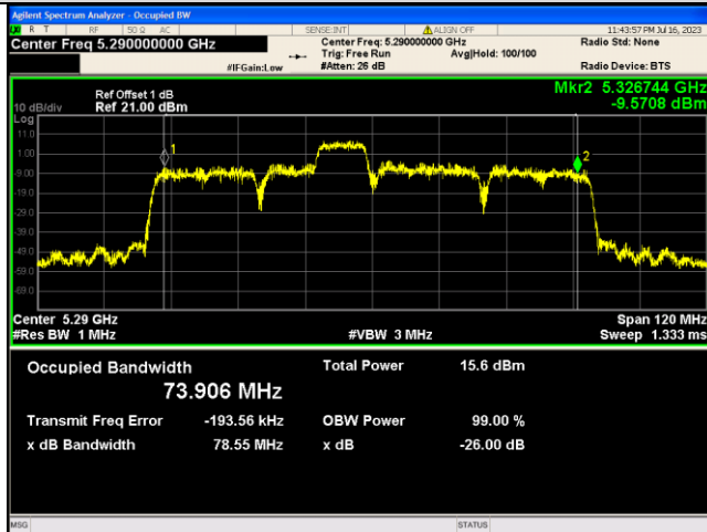
IEEE 802.11ax_Channel 58_80MHz_Antenna 0_RU&amp;Index 106RU56
