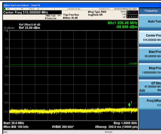
Band4-5MHz-QPSK-20375-1-0-Low-30-1000--59.9-PASS
