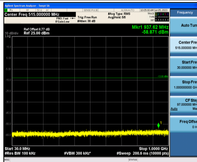
Band4-10MHz-QPSK-20000-1-0-Low-30-1000--58.87-PASS
