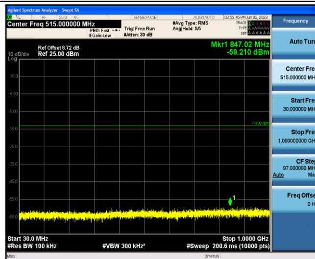
Band2-20MHz-QPSK-18900-1-0-Low-30-1000--59.21-PASS
