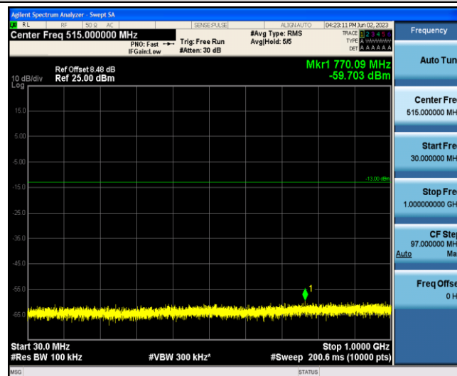
Band4-1.4MHz-QPSK-20175-1-0-Low-30-1000--59.7-PASS
