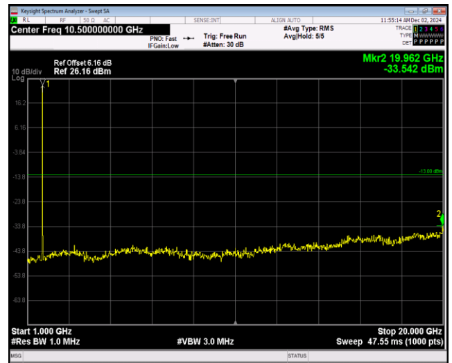
Band4-1.4MHz-QPSK-20175-1RB#0-Range2:1000~20000MHz
