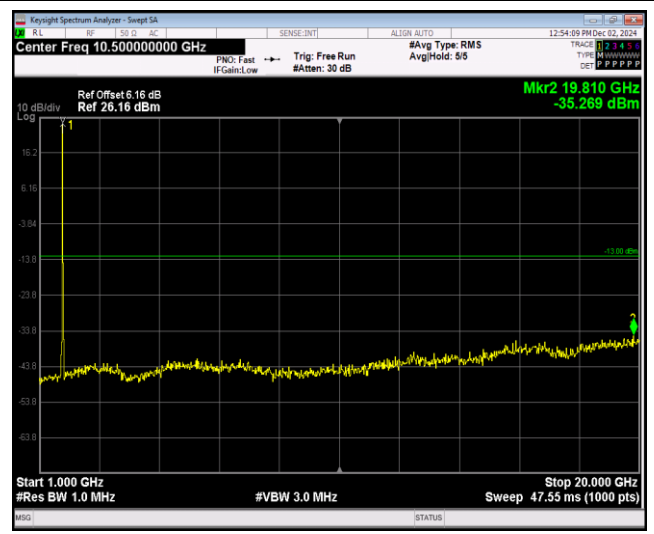
Band4-20MHz-QPSK-20300-1RB#0-Range2:1000~2 0000MHz
