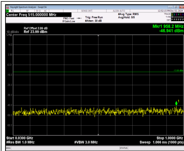
Band4-20MHz-QPSK-20175-1RB#0-Range1:30~100 OMHz
