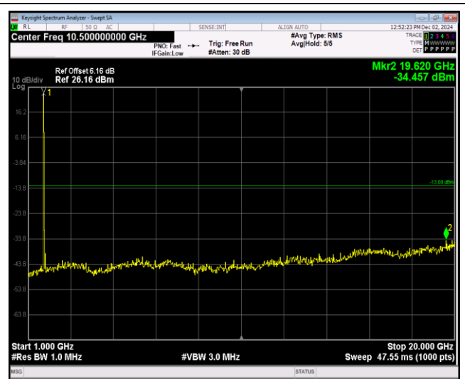
Band4-20MHz-QPSK-20175-1RB#0-Range2:1000~2 0000MHz
