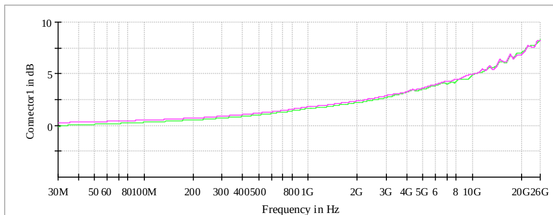
Attenuation
