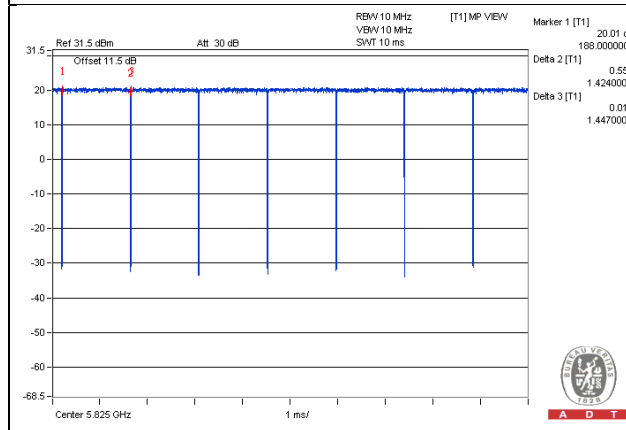
802.11a
