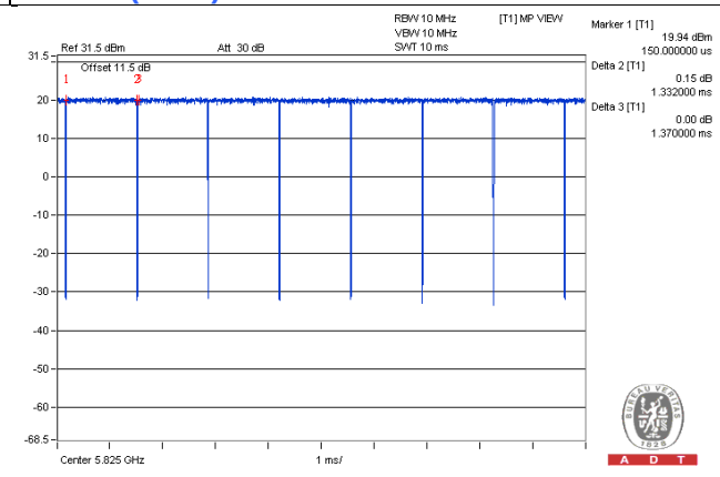
802.11n (HT20)
