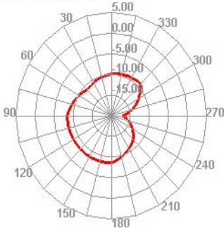
2450.000MHz
