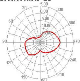
2500.000MHz E2
