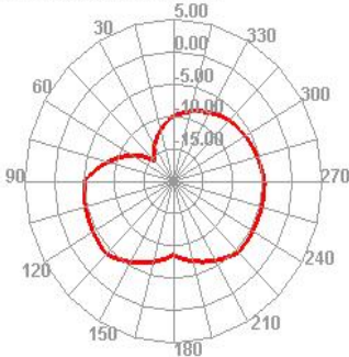
2400.000MHz E2
