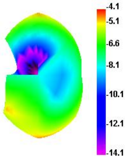
2400.000MHz E1
