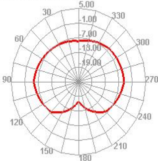
2400.000MHz H
