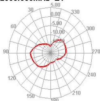
2500.000MHz E1
