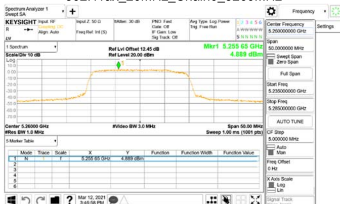
802.11ax_20MHz_Chain0_5260MHz
