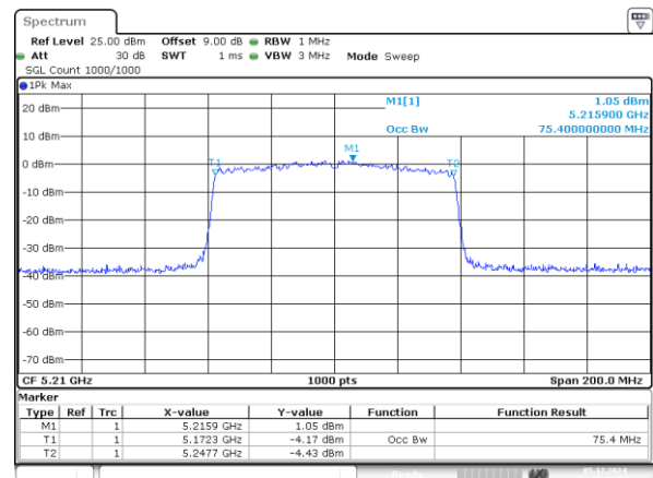
802.11ac80_5210MHz_Chain 1 75.400MHz
