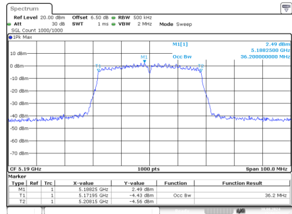
n40_5190MHz_Chain 1 36.200MHz
