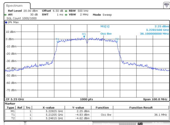
n40_5230MHz_Chain 1 36.100MHz
