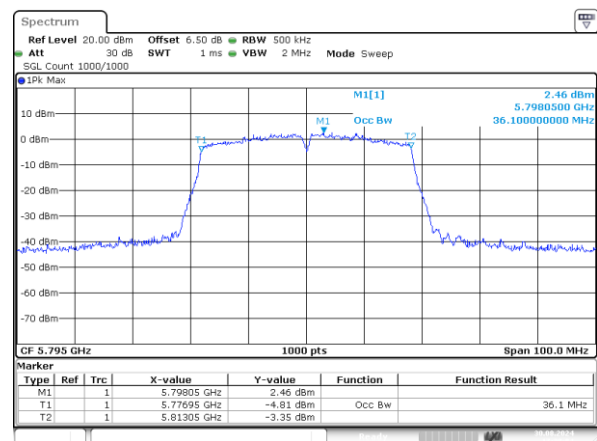
n40_5795MHz_Chain 1 36.100MHz
