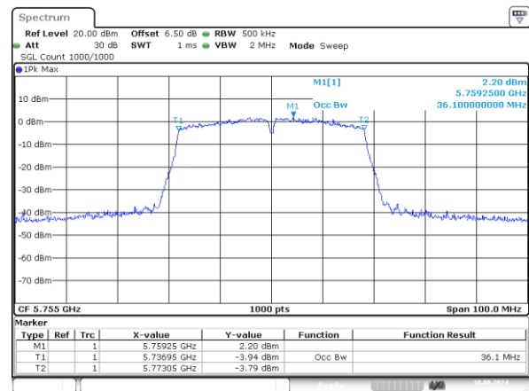
n40_5755MHz_Chain 1 36.100MHz
