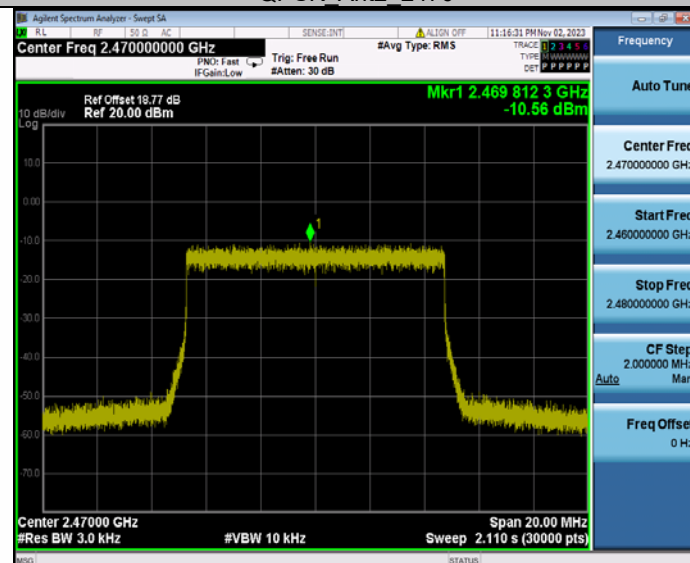
QPSK Ant2 2470
