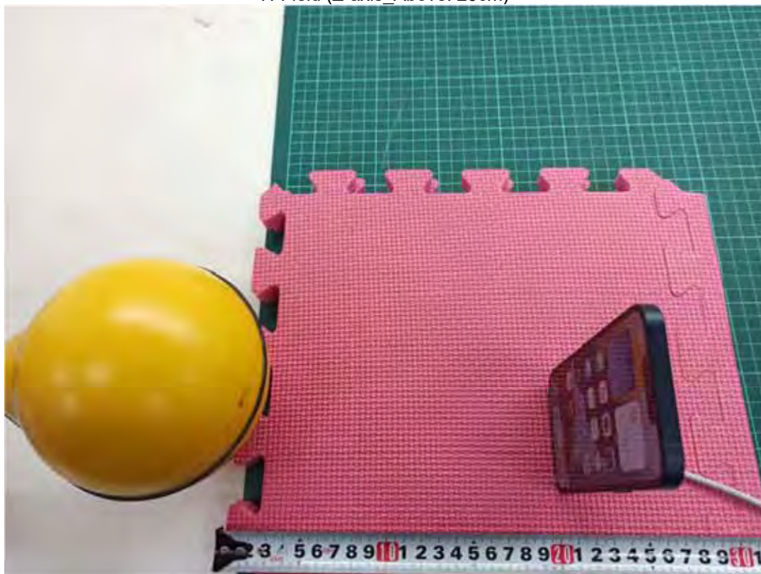
H-Field (Z-axis_Above: 20cm)
