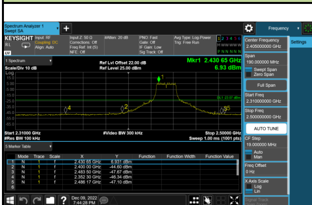
802.11 g CH06 (2437MHz)
