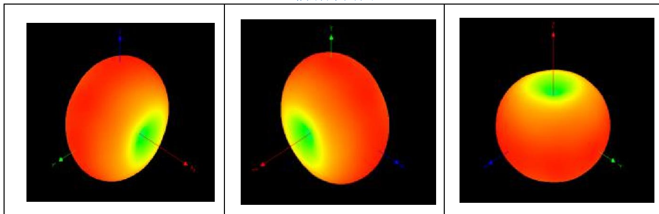
辐射方向图
