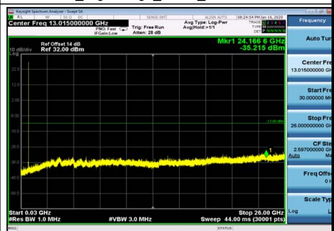
FDD13_HighRange_5MHz_30MHz~26GHz
