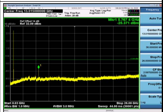
FDD13_HighRange_5MHz_30MHz~26GHz
