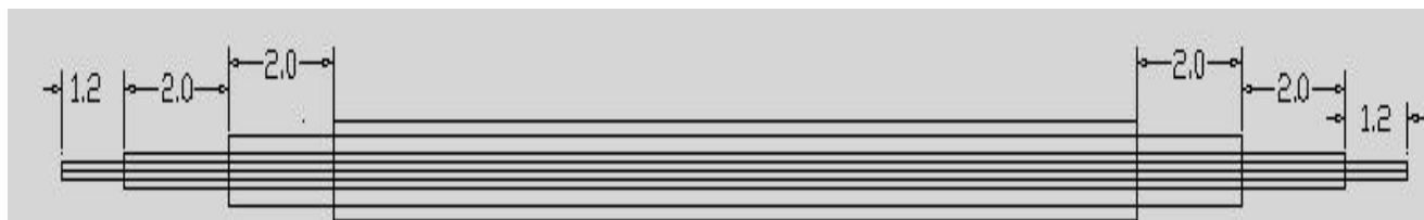
图3 TYY-TX2808-1线长
