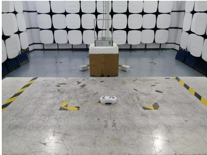
30MHz~1GHz:
