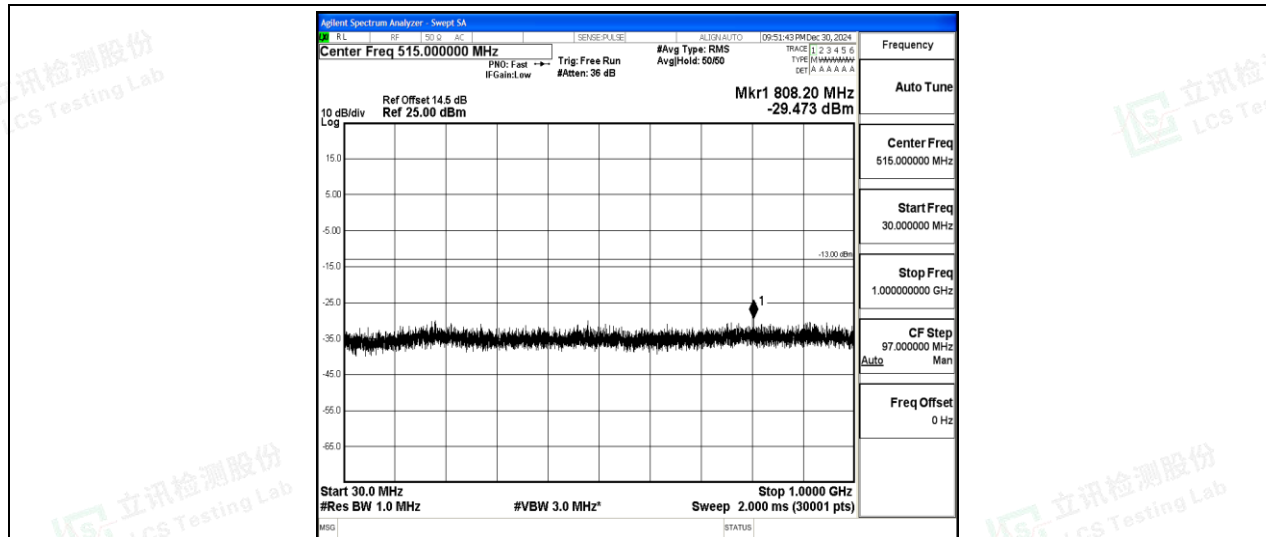
Band2-20MHz-QPSK-18900-1-0-Low-30-1000--29.47-PASS
