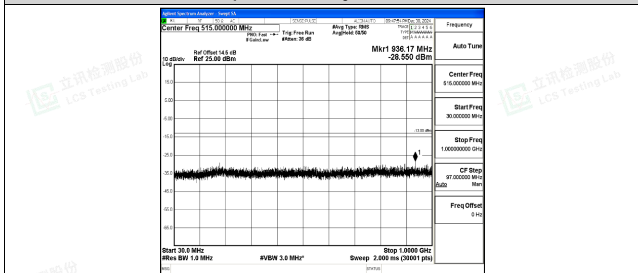
Band2-20MHz-QPSK-18700-1-0-Low-30-1000--28.55-PASS
